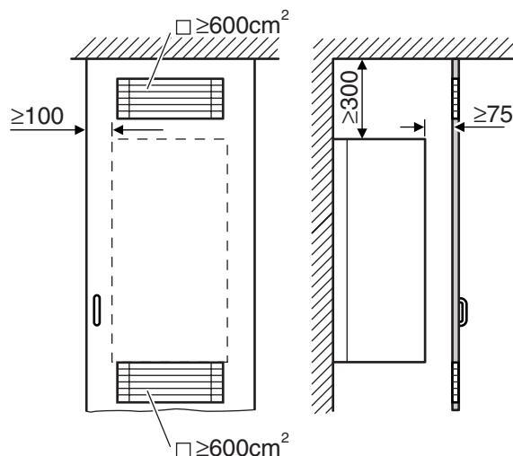
6 720 610 422-04.10
