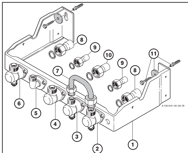
Obr. 11 Montážní připojovací lišta s horizontálními vývody
