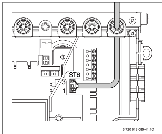
Obr. 26 Připojení termostatu zásobníku
