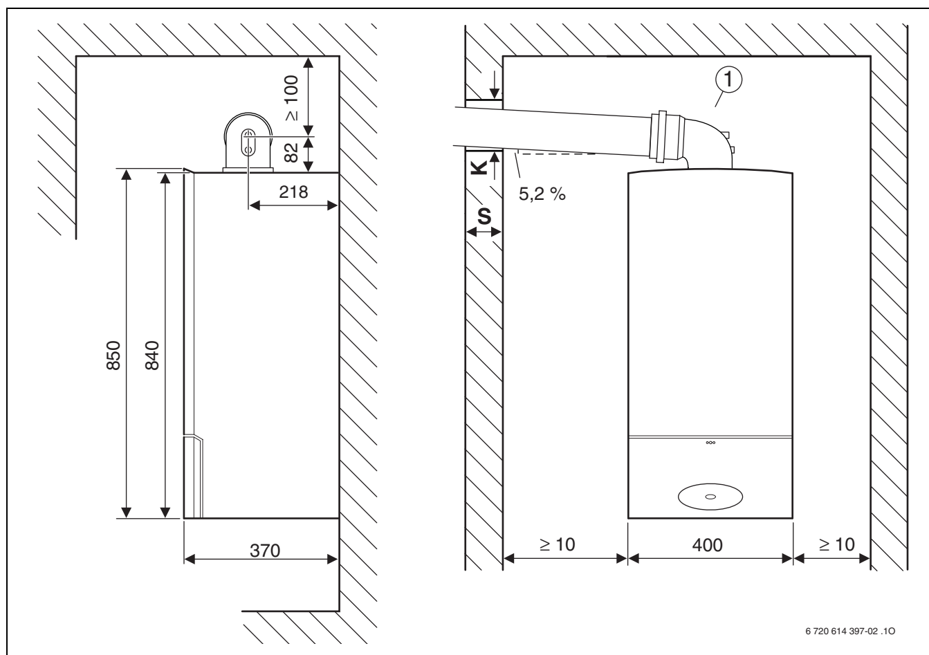
Obr. 6 Odtah spalin Ø 60/100 mm
