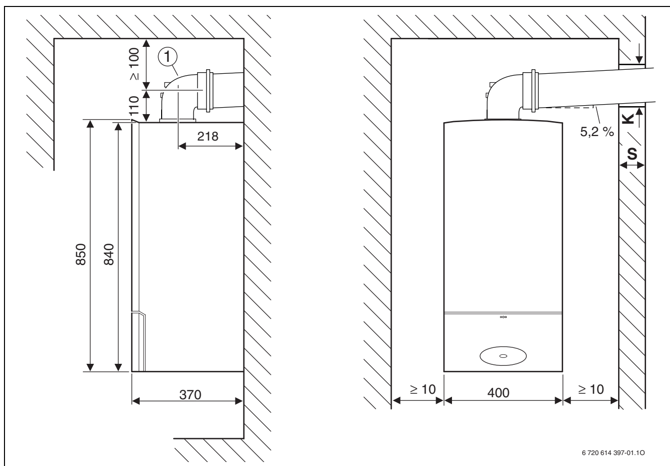
Obr. 5 Odtah spalin Ø 80/125 mm nebo Ø 80 mm
