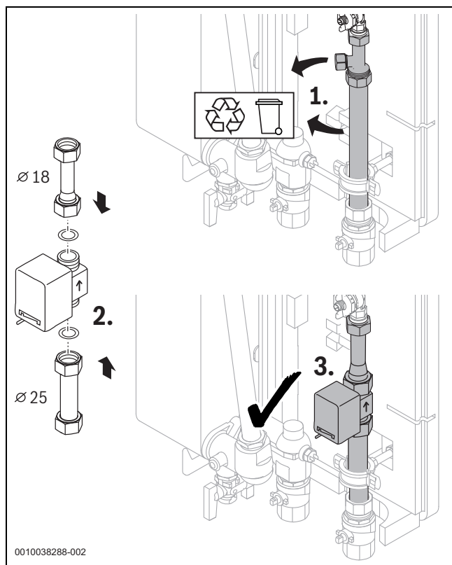
Obr. 25 Montáž kaskádového ventilu (na každou stanici jeden kaskádový ventil)
