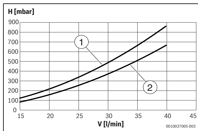
Obr. 9 Tlaková ztráta na sekundární straně stanice pro přípravu teplé vody
