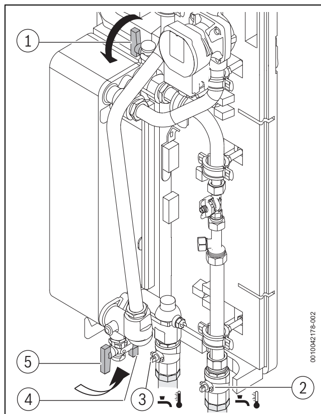
Obr. 56 Vyplachovací/plnicí zařízení na samostatné stanici
