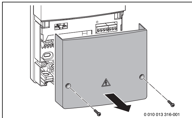
Obr. 46 Otevření modulu
