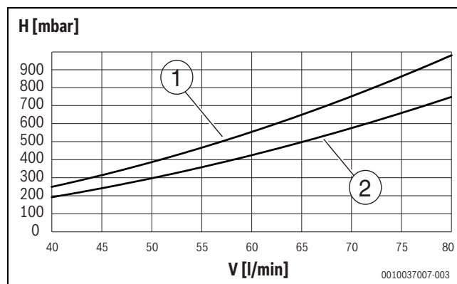
Obr. 11 Tlaková ztráta na sekundární straně kaskády vč. sady potrubního propojení a kaskádového ventilu
