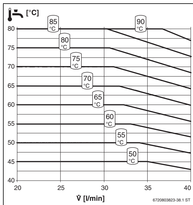
Obr. 58 Chování teploty samostatné stanice FF40S
