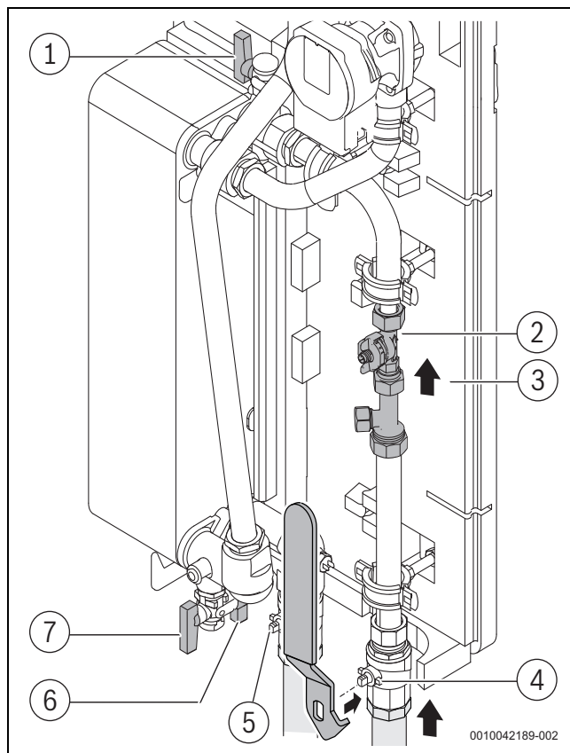
Obr. 65 Výměna průtokového čidla
