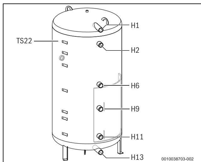
Obr. 36 Akumulační zásobník jako solární zásobník (oddělený objem), hydraulika (→ obrázek 6, strana 7)
