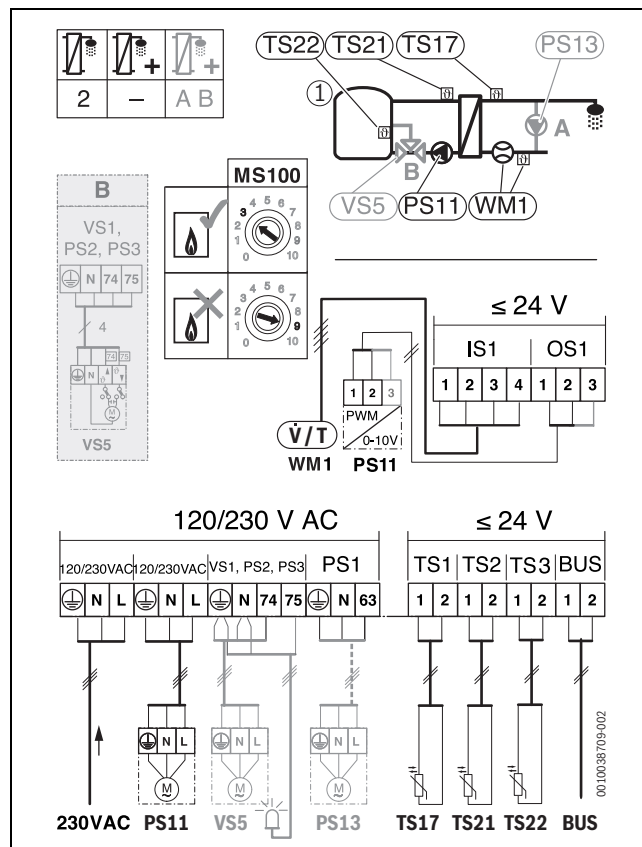
Obr. 47 Připojovací svorky u stanice pro přípravu teplé vody (samostatná stanice)
