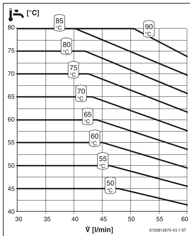
Obr. 59 Chování teploty kaskády FF54S
