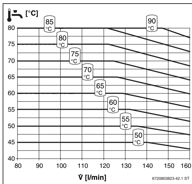
Obr. 62 Chování teploty kaskády FF160S
