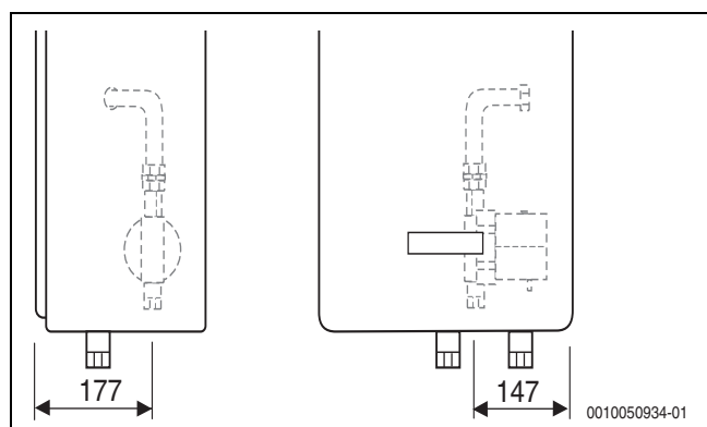
Obr. 14 Rozměry cirkulační větve (příslušenství)
