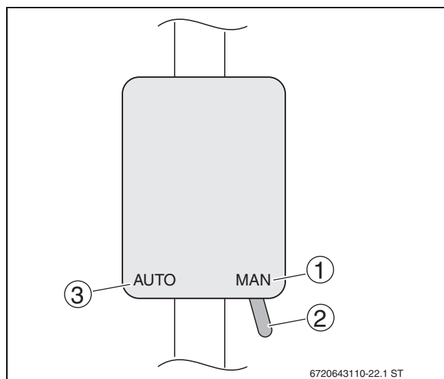
Obr. 55 Nastavení 2cestného motoricky řízeného ventilu do polohy "MAN" pro plnění a vyplachování
