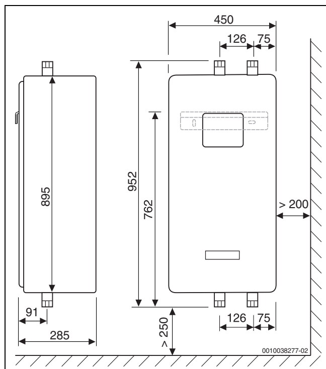
Obr. 13 Rozměry samostatné stanice v mm (nástěnný držák znázorněn šedě)
