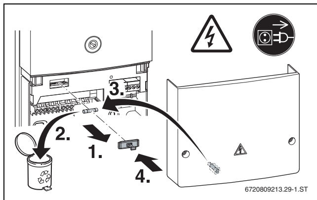
Obr. 66 Výměna pojistky
