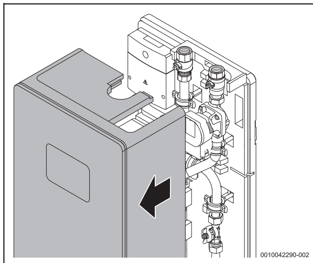
Obr. 1 Odstranění přední tepelné izolace
