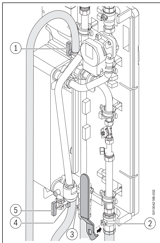
Obr. 64 Údržba stanice pro přípravu teplé vody
