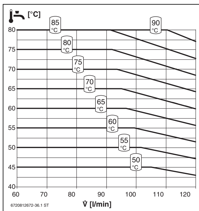
Obr. 61 Chování teploty kaskády FF120S
