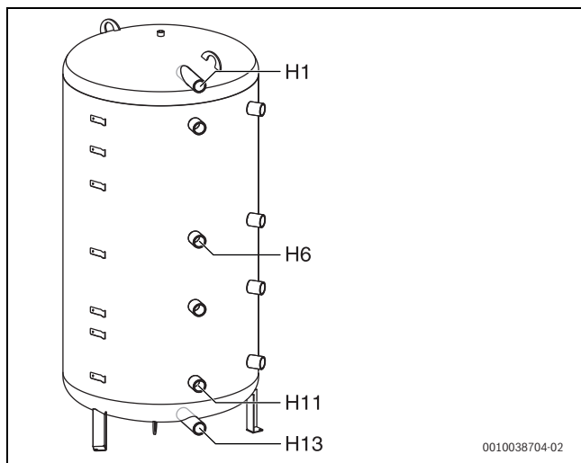
Obr. 37 Akumulační zásobník jako solární zásobník pro přehřívací systém (lze i s interním výměníkem tepla), hydraulika (→ obrázek 7, strana 8)
