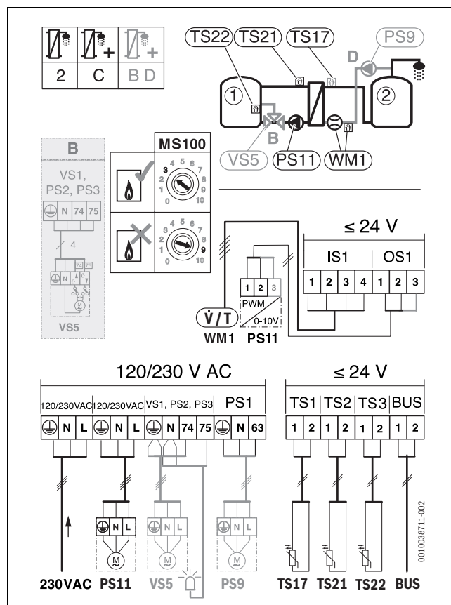
Obr. 48 Připojovací svorky u předehřívací stanice pro přípravu teplé vody
