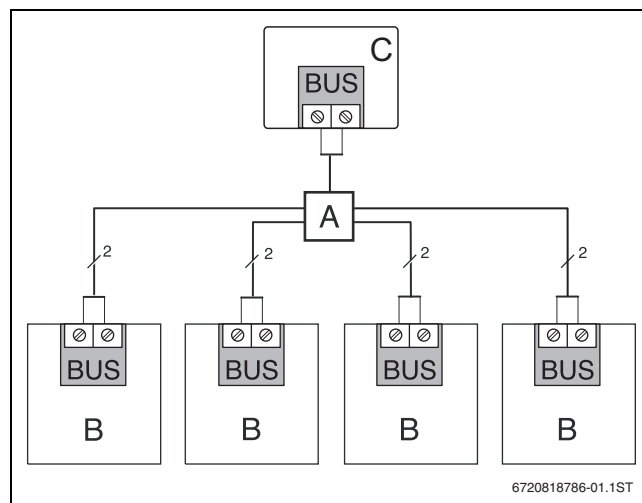
Obr. 54 Připojení sběrnových kabelů
