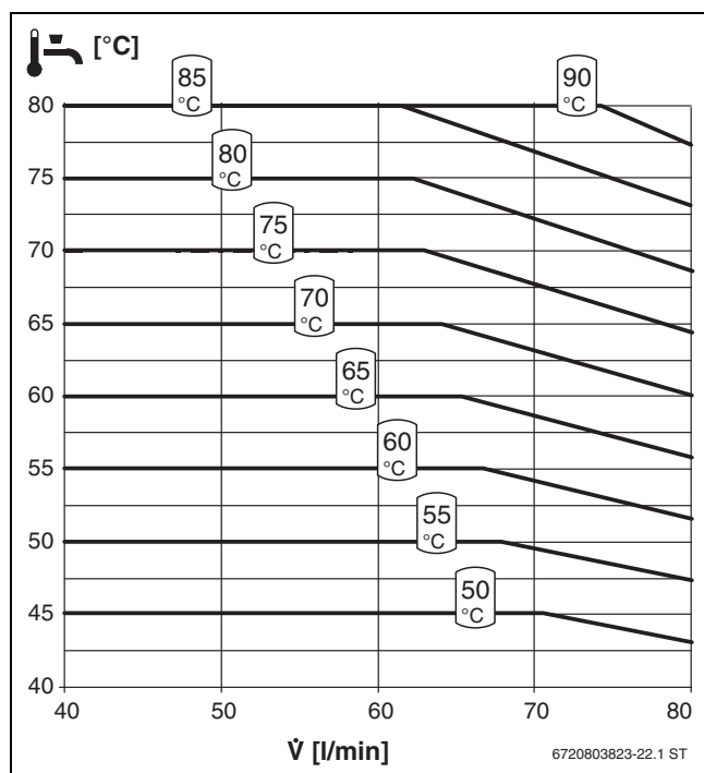
Obr. 60 Chování teploty kaskády FF80S
