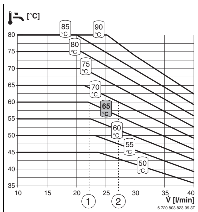
Obr. 57 Chování teploty samostatné stanice FF27S
