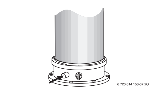
Obr. 53 Sejmутí zásepky
