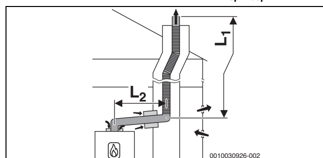
Obr. 21 Pružné potrubí vedení odtahu spalin v šachtě podle B 23p /B 53p s přívodem vzduchu závislým na vzduchu z prostoru na zařízení a koaxiálním spojovacím dílem mezi místem instalace a šachtou
