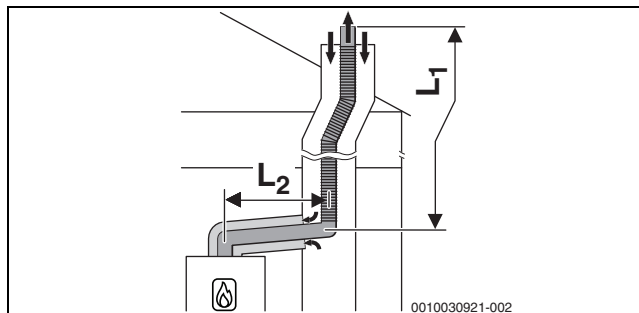
Obr. 19 Flexibilní potrubí odtahu spalin podle C 93x v šachtě a koaxiální systém odvodu spalin v místě instalace
