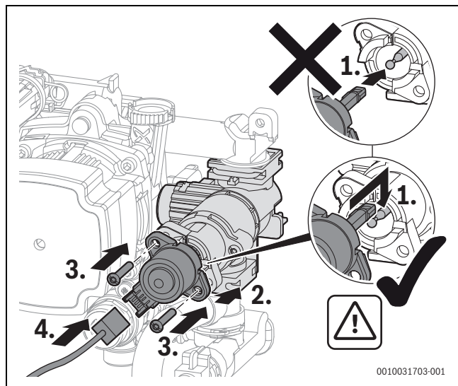
Obr. 89 Namontování motoru 3cestného ventilu (varianata se šrouby)
