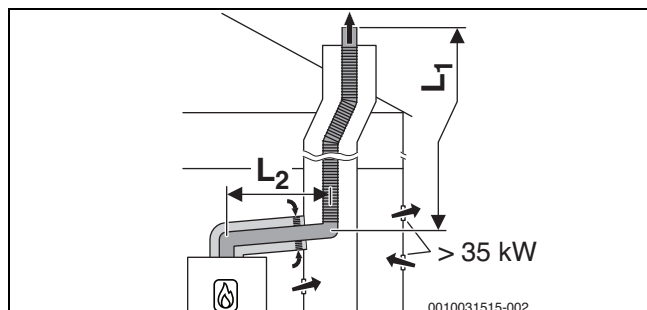
Obr. 23 Pružné potrubí vedení odtahu spalin v šachtě podle B 33 s přívodem vzduchu závislým na vzduchu z prostoru koaxiálním systémem odvodu spalin v místě instalace
