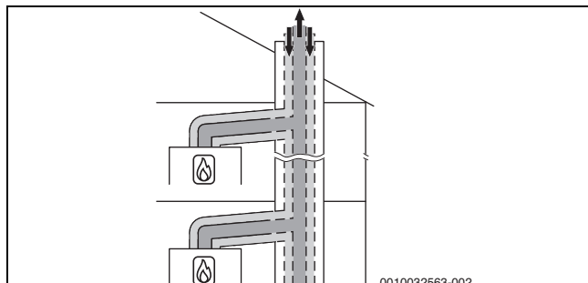
Obr. 24 Zapojení několika tepelných zdrojů do jednoho spalinového zařízení podle C_{(10)3x} pomocí koaxiálního systému odvodu spalin v místě instalace
