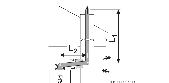
Obr. 20 Pevné vedení odtahu spalin v šachtě podle B 23p /B 53p s přívodem vzduchu závislým na vzduchu z prostoru na zařízení a koaxiálním spojovacím dílem mezi místem instalace a šachtou
