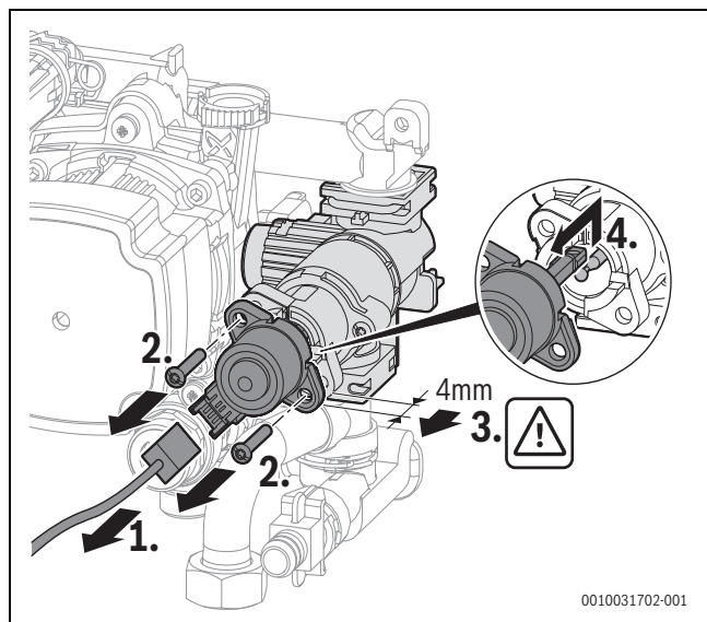
Obr. 88 Vymontování motoru 3cestného ventilu (varianata se šrouby)
