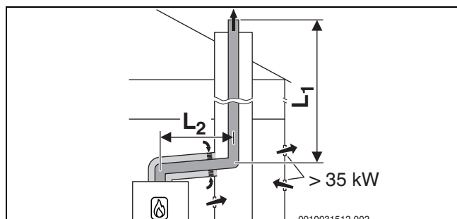
Obr. 22 Pevné vedení odtahu spalin v šachtě podle B 33 s přívodem vzduchu závislým na vzduchu z prostoru koaxiálním systémem odvodu spalin v místě instalace
