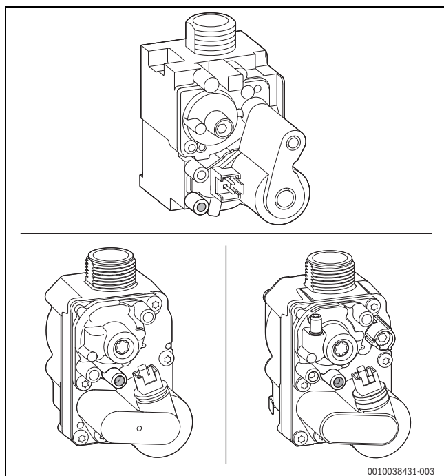
Obr. 50 Nahoře a dole vlevo: Nenastavitelný plynový ventil, dole vpravo: Nastavitelný plynový ventil
