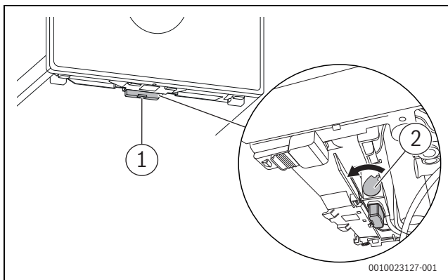
Obr. 5 Zajištění Key
