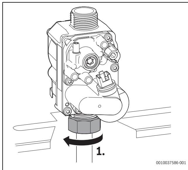
Obr. 149 Povolení převlečné matice
