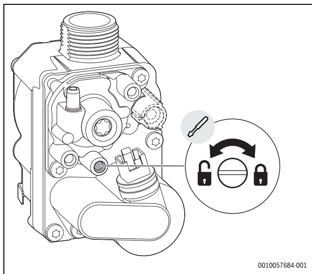
Obr. 113 Měření připojovacího tlaku plynu
