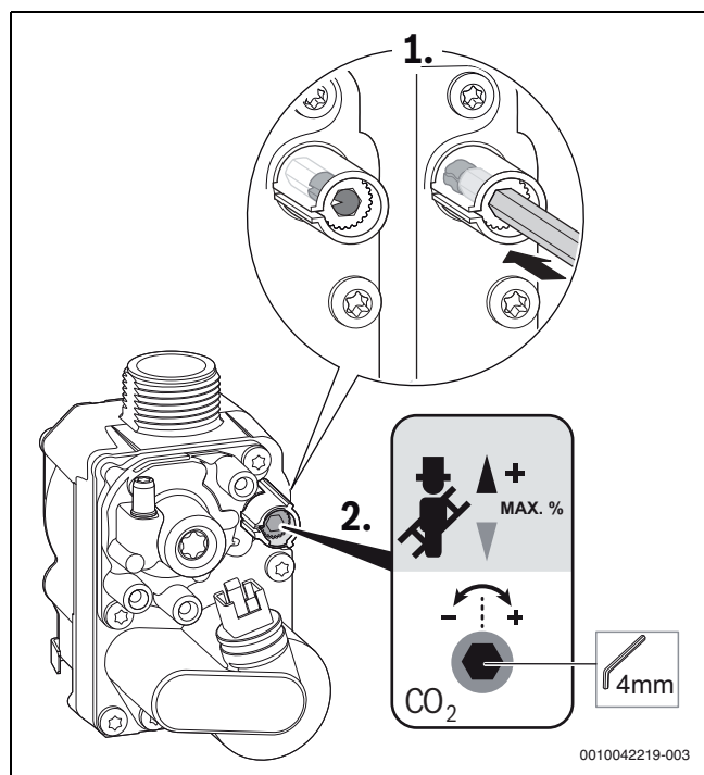
Obr. 115 Nastavení obsahu CO 2 /O 2 při maximálním jmenovitém tepelném výkonu
