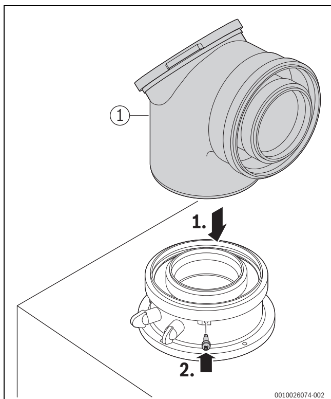
Obr. 81 Nasazení dílu systému odvodu spalin a zajištění šroubem
