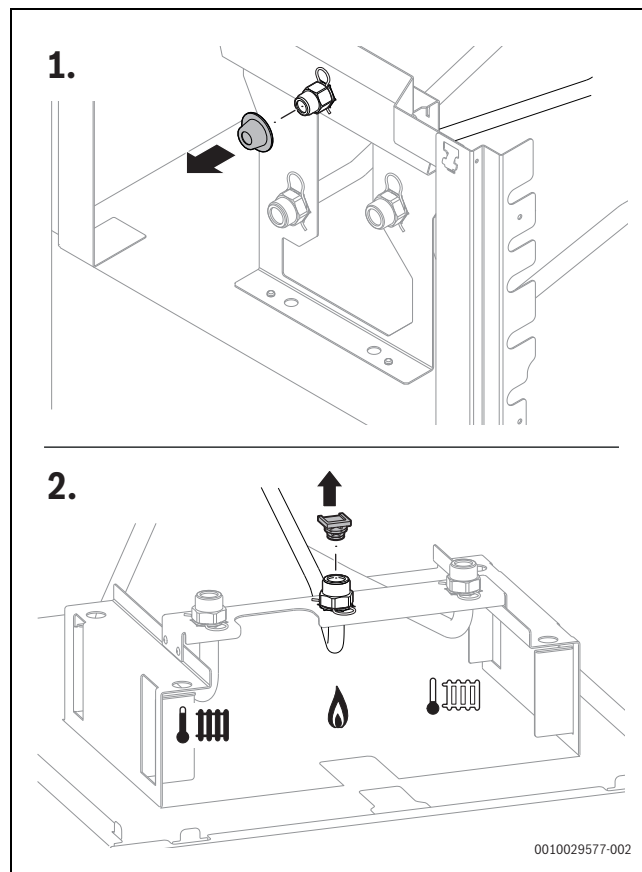
Obr. 59 Sejmutí krytky a záslepký z plynového potrubí
