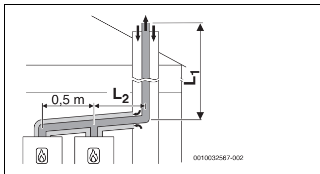
Obr. 44 Kaskáda se 2 zařízeními: Pevná spalínová cesta podle C_{93x} v šachtě a koaxiální systém odvodu spalin v místě instalace
