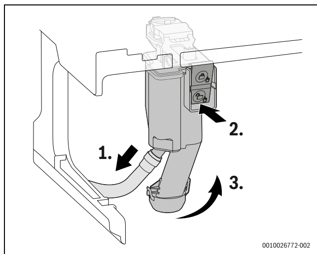
Obr. 156 Vymontování sifonu kondenzátu
