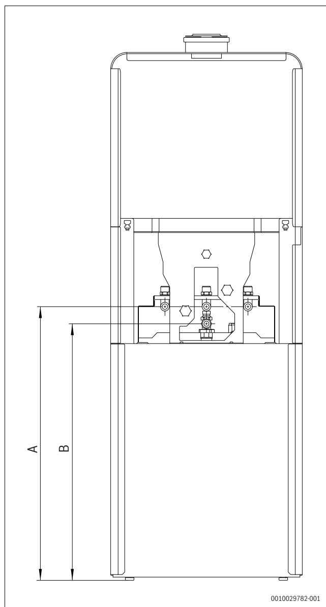
Obr. 18 Pohled ze zadní strany (rozměry v mm)
