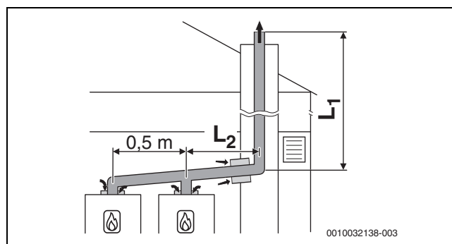
Obr. 43 Kaskáda se 2 zařízeními: Pevné vedení odtahu spalin v šachtě podle B 53P s přívodem vzduchu závislým na vzduchu z prostoru na zařízení
