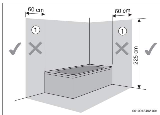
Obr. 45 Ochranné úseky
