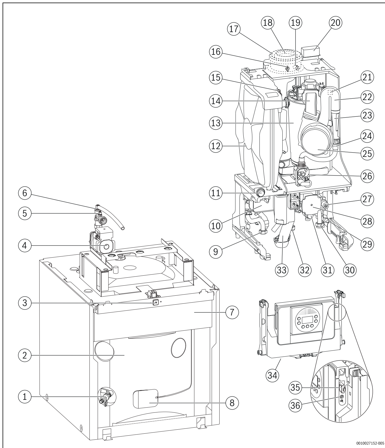
Obr. 5 Přehled výrobku
