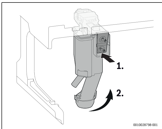
Obr. 68 Vyjmutí sifonu kondenzátu
