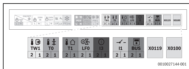
Obr. 95 Úsek nízkého napětí: svorkovnice
