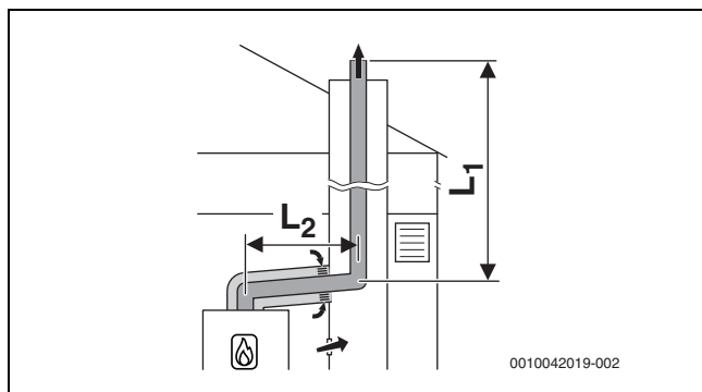
Obr. 36 Pevné vedení odvodu spalin v šachtě podle B 53p s přívodem vzduchu závislým na vzduchu z prostoru koaxiálním systémem odvodu spalin v místě instalace
