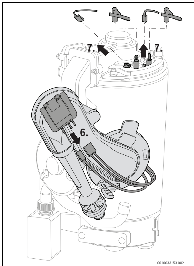
Obr. 128 Odpojení kabelů
