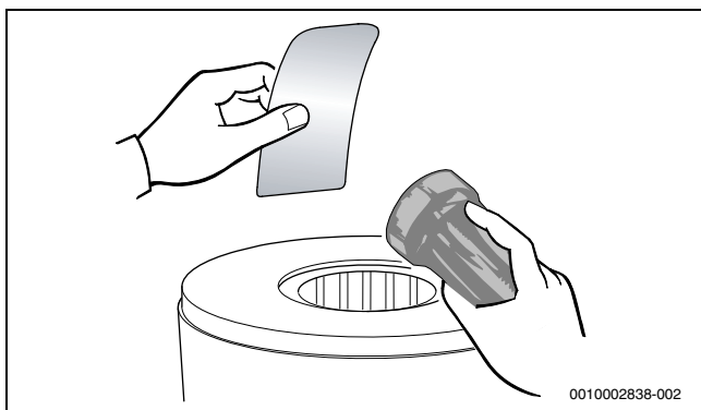
Obr. 139 Kontrola zbytků v tepelném výměníku
