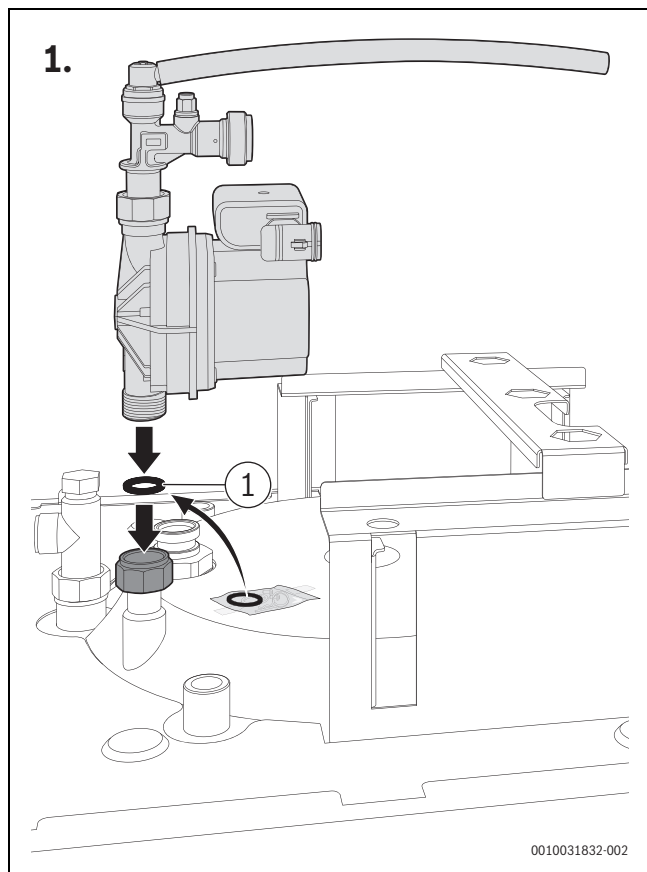
Obr. 53 Vsazení nabíjecího čerpadla stratifikačního zásobníku
