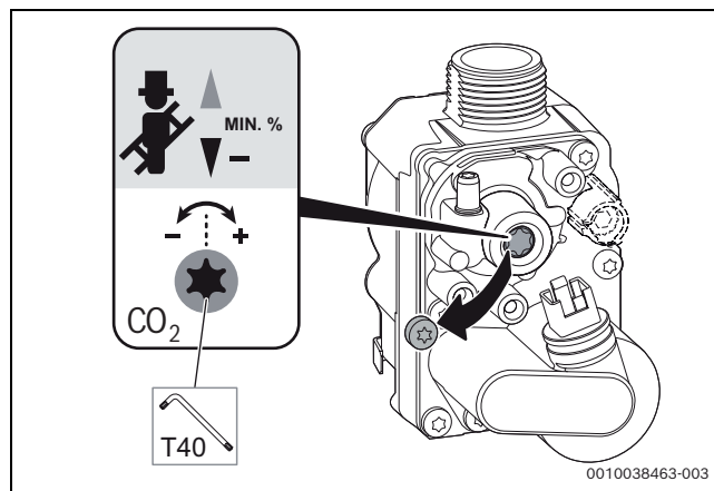
Obr. 116 Nastavení obsahu CO 2 /O 2 při minimálním jmenovitém tepelném výkonu
