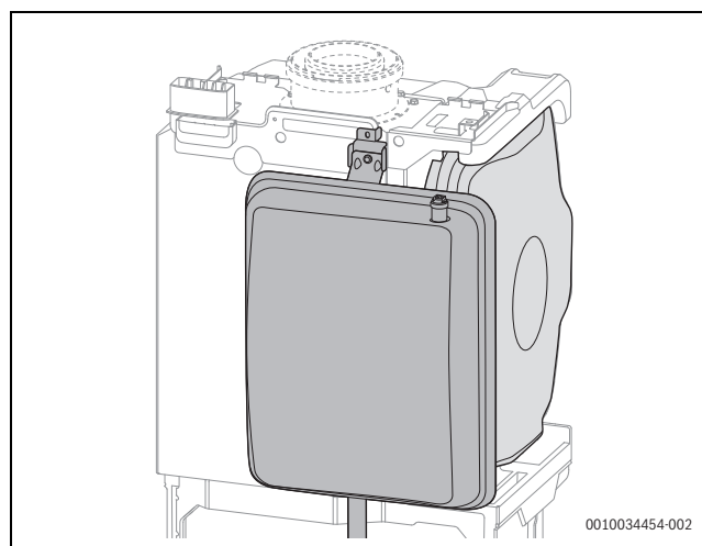
Obr. 49 2 expanzní nádoby instalované do zařízení
