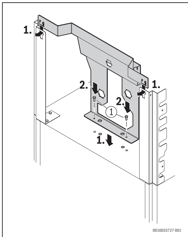
Obr. 56 Montáž Základním modulem (příslušenství CS 35) – krok 2
