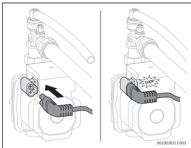
Obr. 96 Elektrické připojení nabíjecího čerpadla stratifikačního zásobníku
