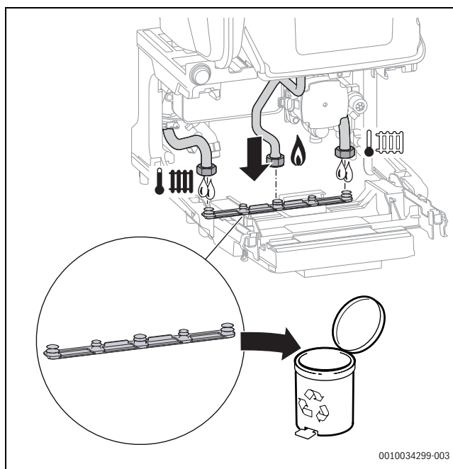
Obr. 64 Vyjmutí krycí lišty ze zařízení
