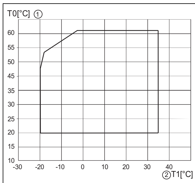
Obr. 20 Tepelné čerpadlo bez dotopu
