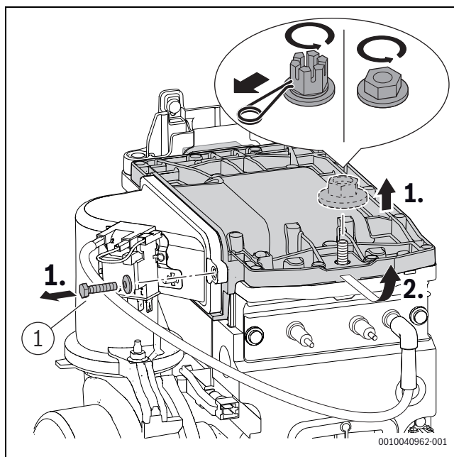
Obr. 50 Odmontování krytu hořáku
