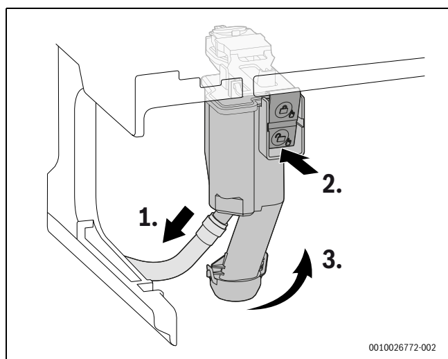
Obr. 63 Vymontování sifonu kondenzátu
