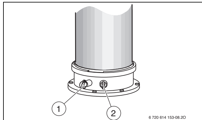
Obr. 47 Měřící hrdlo spalin a měřící hrdlo spalovacího vzduchu
