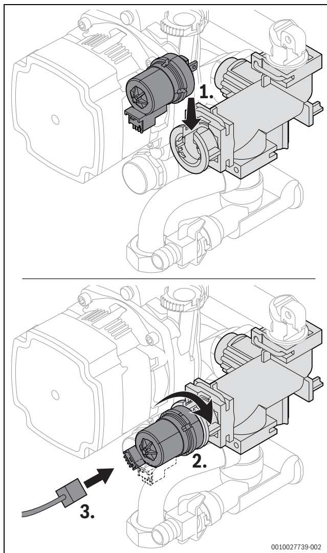
Obr. 71 Namontování motoru 3cestného ventilu (varianta bez šroubů)
