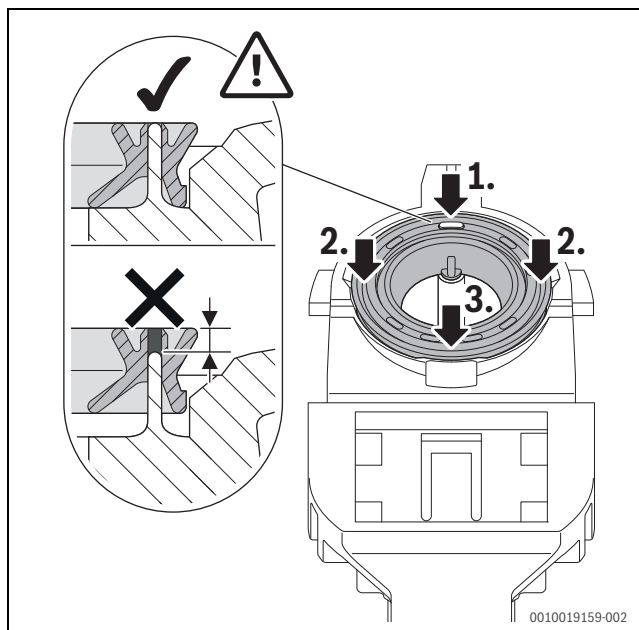
Obr. 65 Přitlačení těsnění
