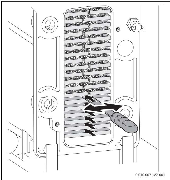
Obr. 59 Čisticí nůž
