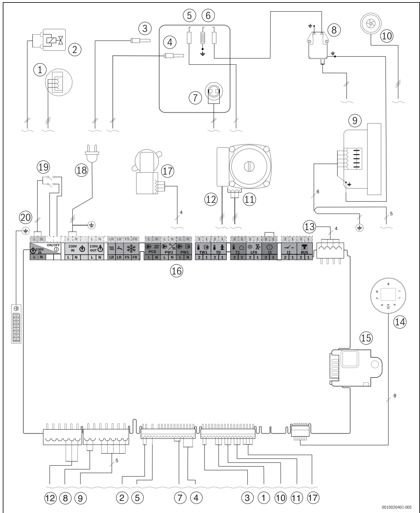
Obr. 75 Elektrické kabelové propojení
