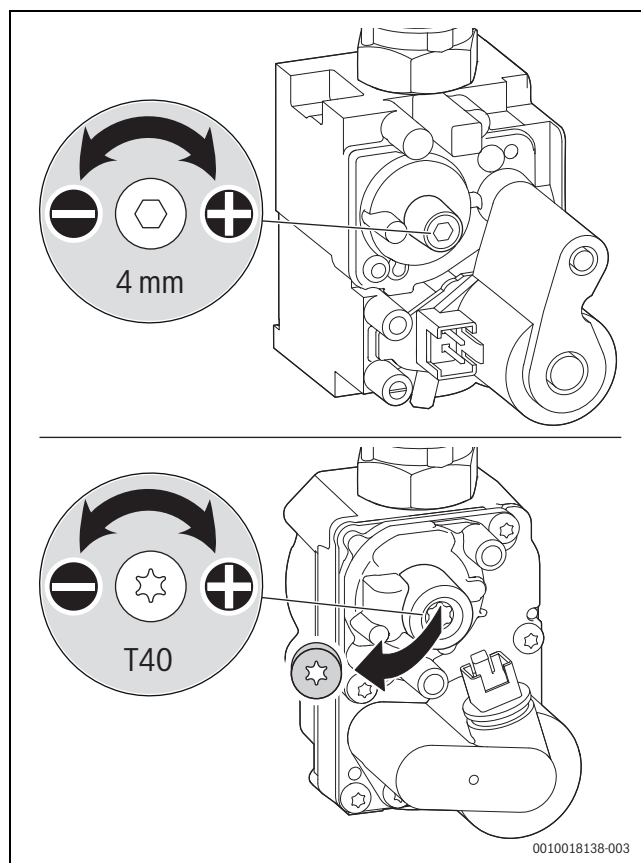
Obr. 45 Nastavení obsahu CO 2 nebo O 2
