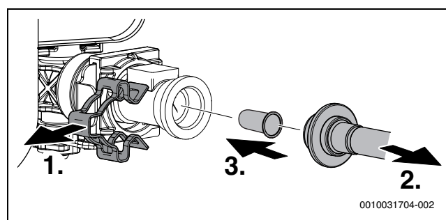
Obr. 55 Vytážení sítka z potrubí studené vody
