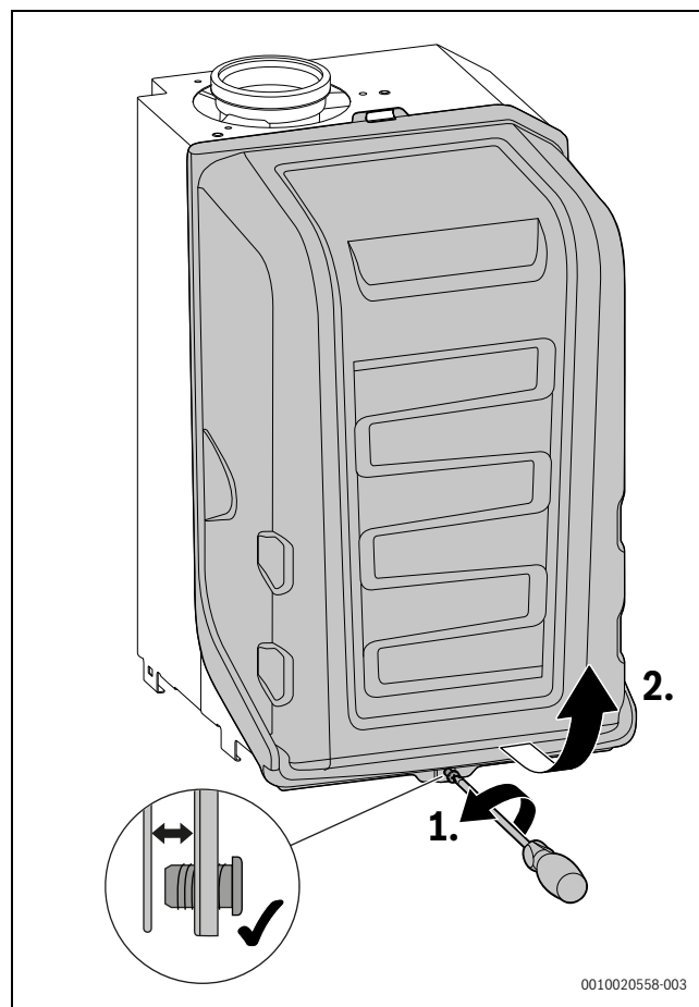
Obr. 42 Sejmutí krytu hořáku
