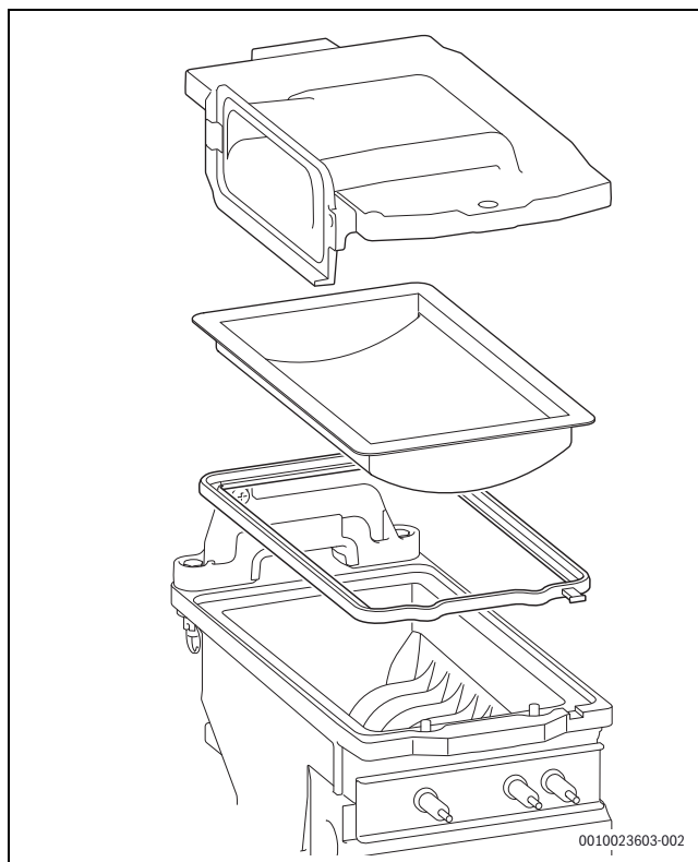
Obr. 51 Hořák
