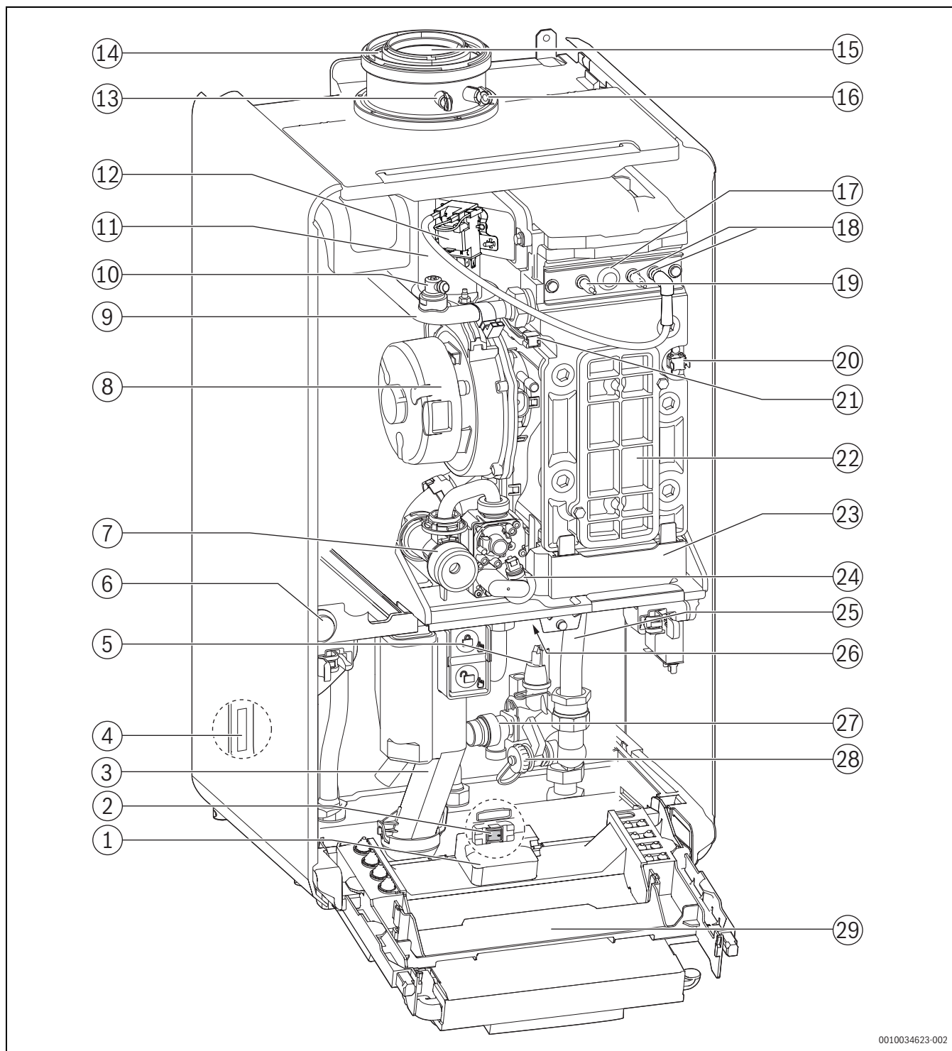
Obr. 4 Přehled výrobku
