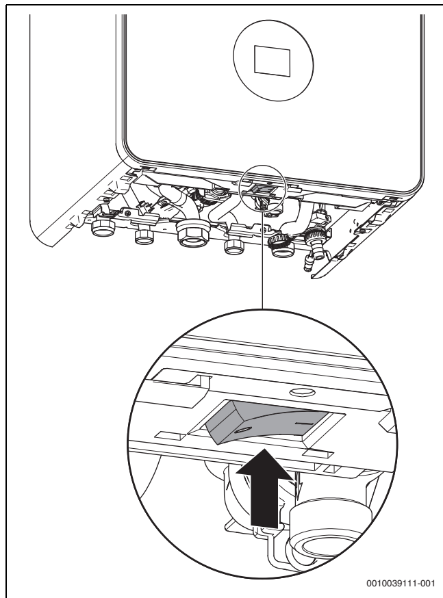
Obr. 1 Hlavní vypínač
