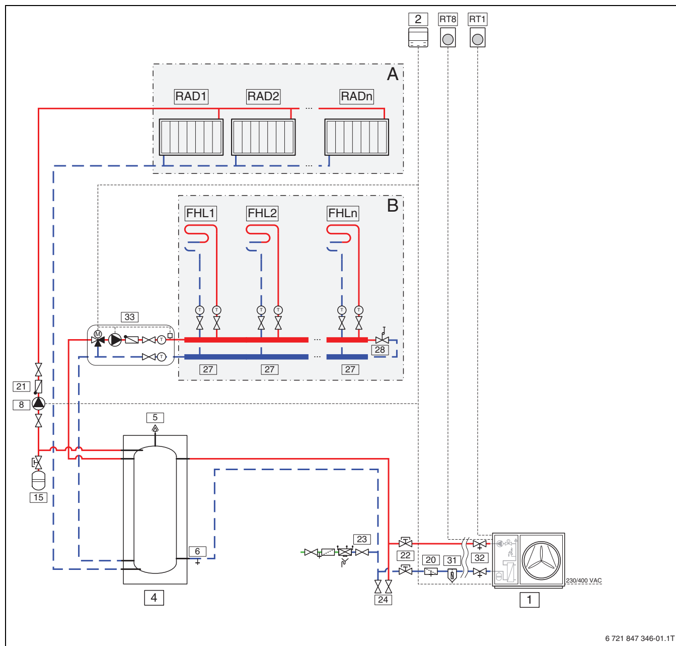
Obr. 18 Venkovní jednotka s nejméně jedním otopným okruhem, podlahovým vytápěním a otopnými tělesy (CS2000AWF 4-6 R-S, CS2000AWF 8-10 R-S, CS2000AWF 12-16 R-S/T)
