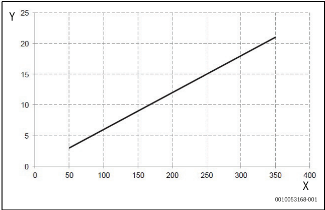
Obr. 56 Celkový objem pro expanzní nádrž (velikosti CS2000AWF 4 R-S až CS2000AWF 16 R-S/CS2000AWF 16 R-T)
