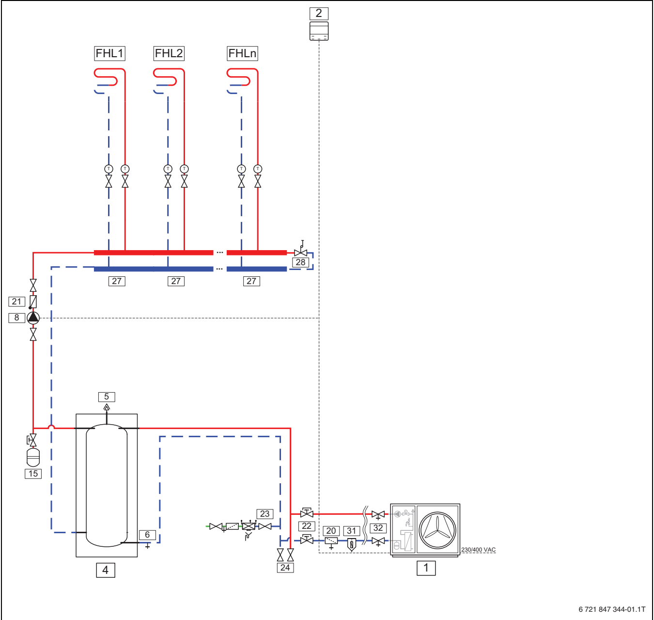
Obr. 16 Venkovní jednotka s nejméně jedním otopným okruhem (CS2000AWF 4-6 R-S, CS2000AWF 8-10 R-S, CS2000AWF 12-16 R-S/T)
