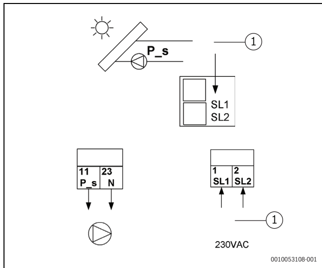
Obr. 76 Konfigurace soláru/solárního čerpadla na rozhraní HMI
