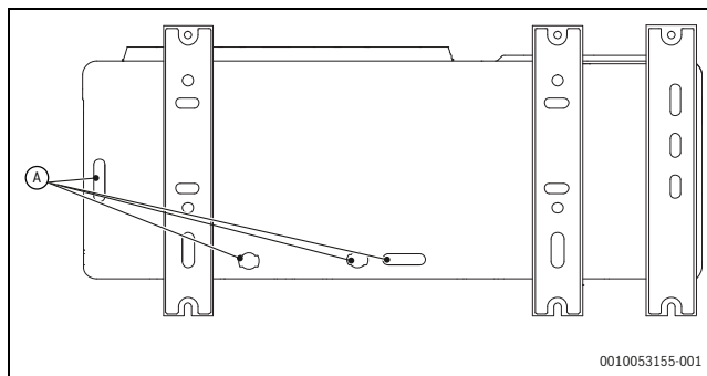
Obr. 47 Odtokové otvory
