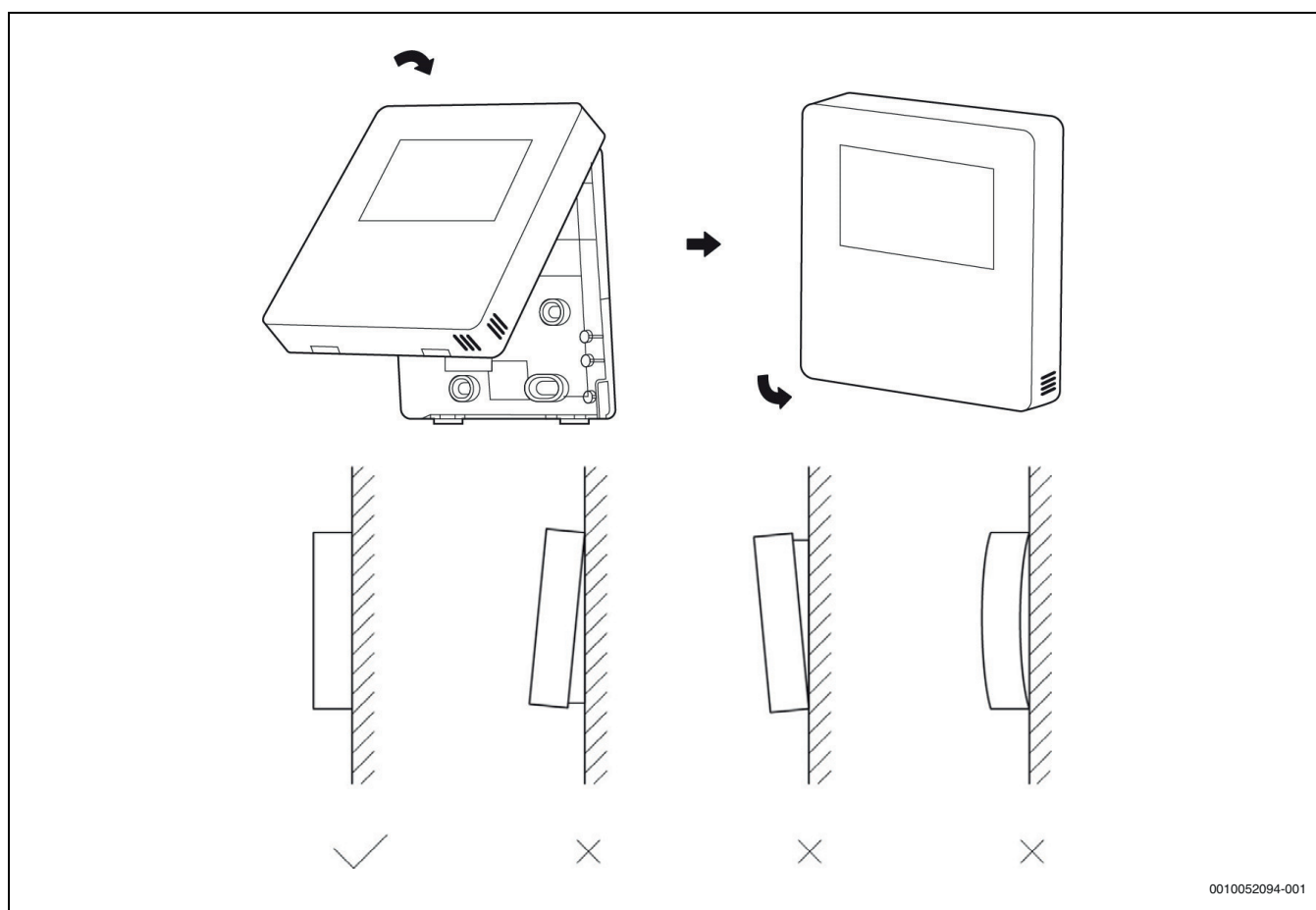
Obr. 100 Instalace předního krytu
