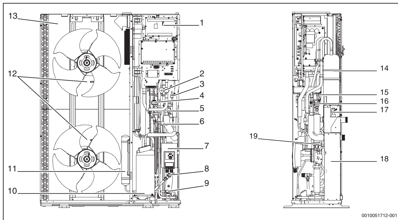
Obr. 5 Velikosti CS2000AWF 18 R-T až CS2000AWF 30 R-T
