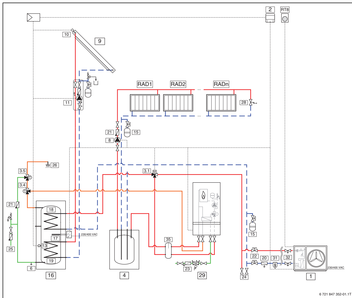
Obr. 22 Venkovní jednotka s nejméně jedním otopným okruhem, externím přídavným ohřívačem, zásobníkem TV a solárem (CS2000AWF 4-6 R-S, CS2000AWF 8-10 R-S, CS2000AWF 12-16 R-S/T)
