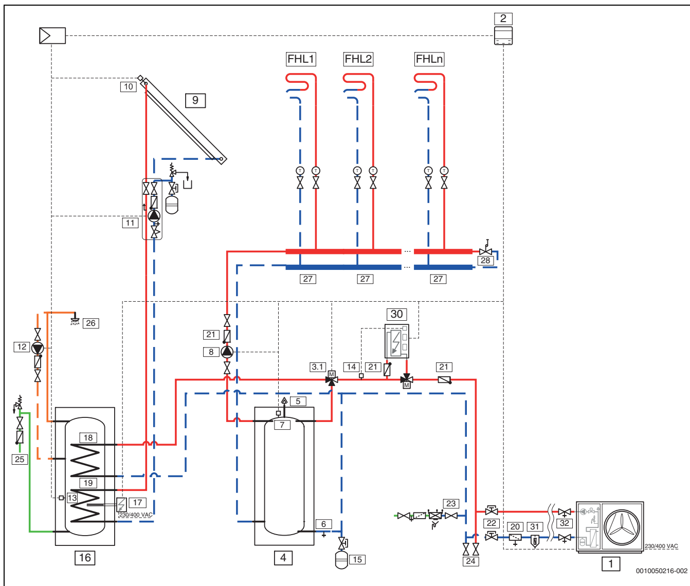
Obr. 15 Venkovní jednotka s nejméně jedním otopným okruhem, záložním elektrickým ohřeváčem, zásobníkem TV a solárem (CS2000AWF 4-6 R-S, CS2000AWF 8-10 R-S, CS2000AWF 12-16 R-S/T)
