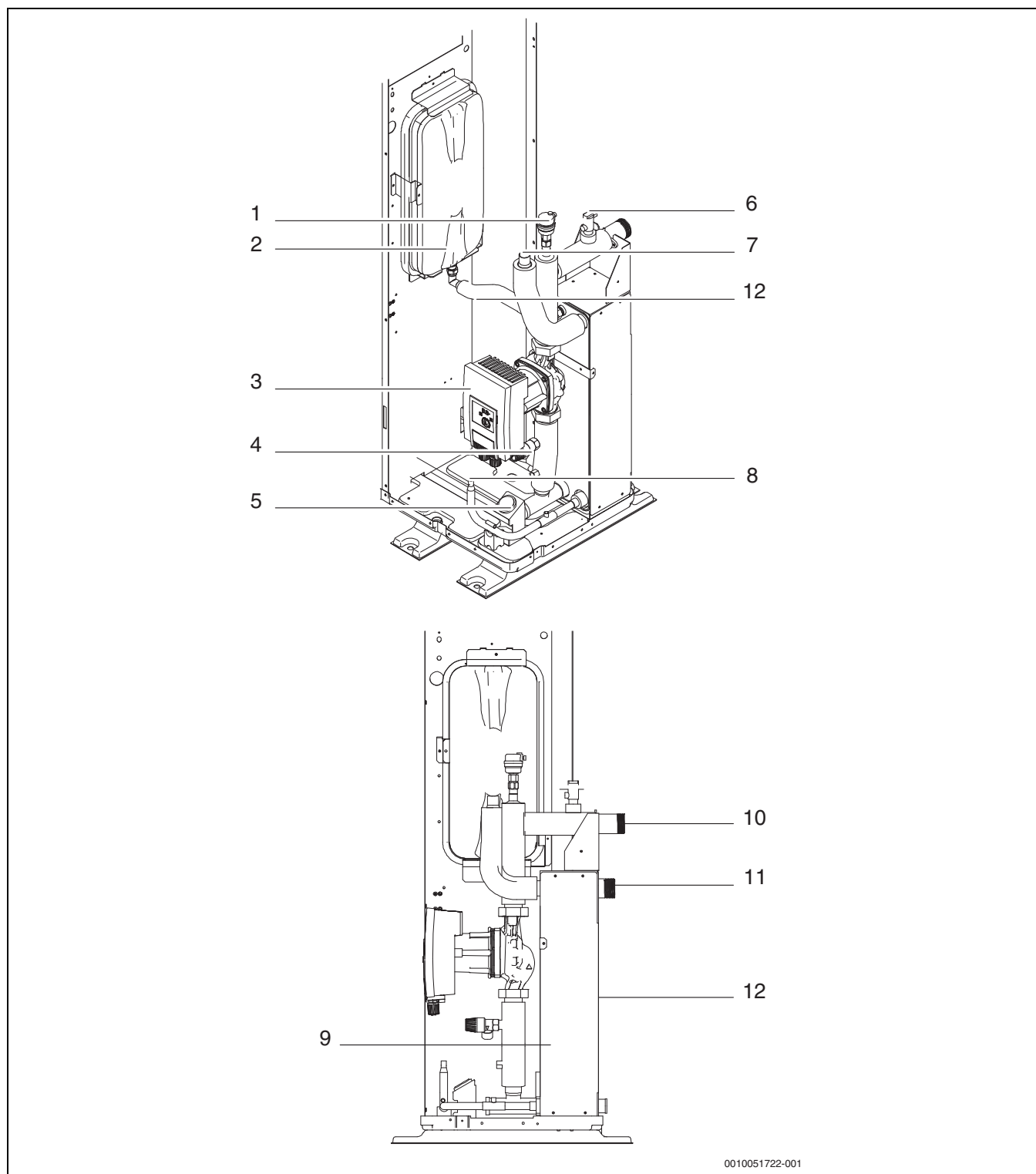
Obr. 8 Velikosti CS2000AWF 18 R-T až CS2000AWF 30 R-T
