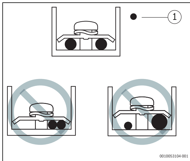
Obr. 70 Nebezpečí přehřátí v důsledku uvolněných vodičů
