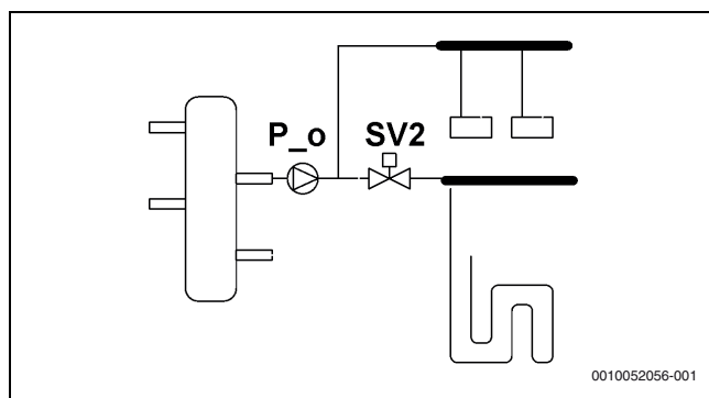
Obr. 81 Dvouzónová soustava
