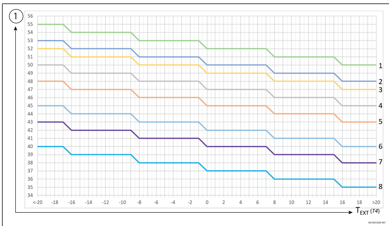
Obr. 146 Režim Vytápění v soustavách s terminálovou distribucí
