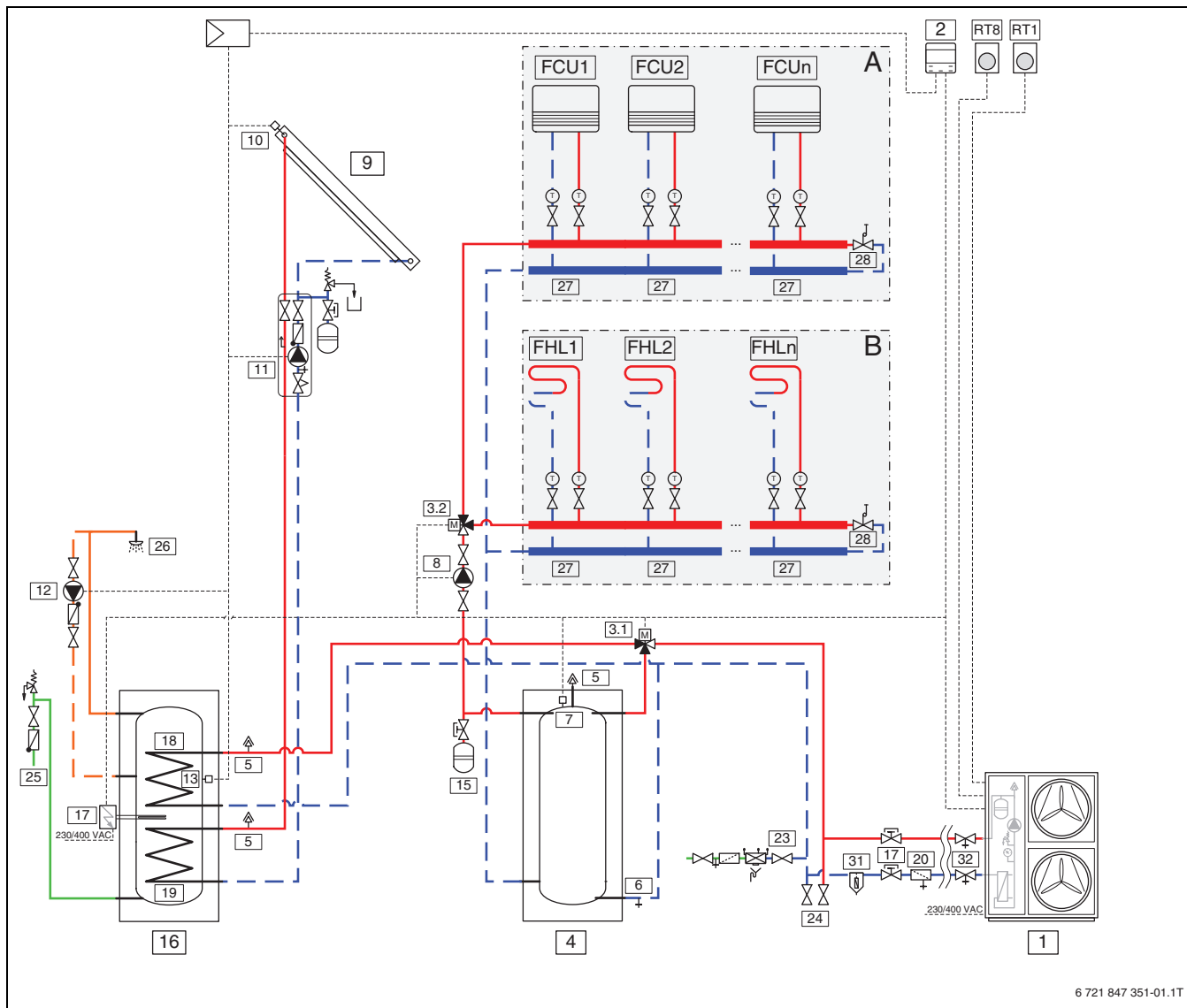
Obr. 21 Venkovní jednotka s nejméně jedním topným okruhem, záložním elektrickým ohřívačem, zásobníkem TV a solárem (CS2000AWF 18 -30 R-T)
