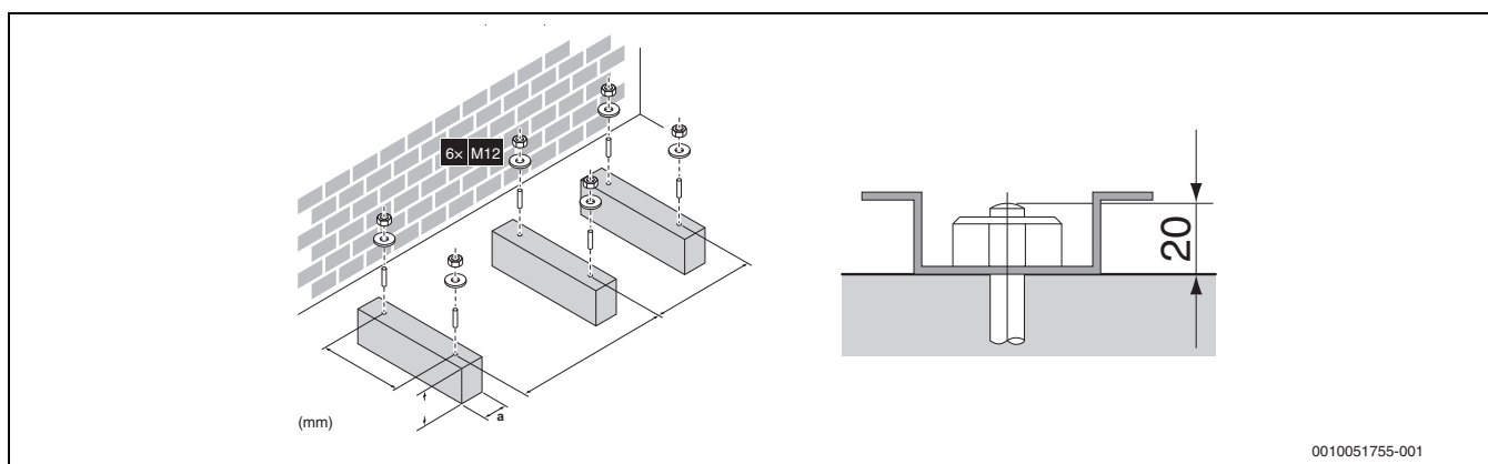
Obr. 41 Přízemní montáž
