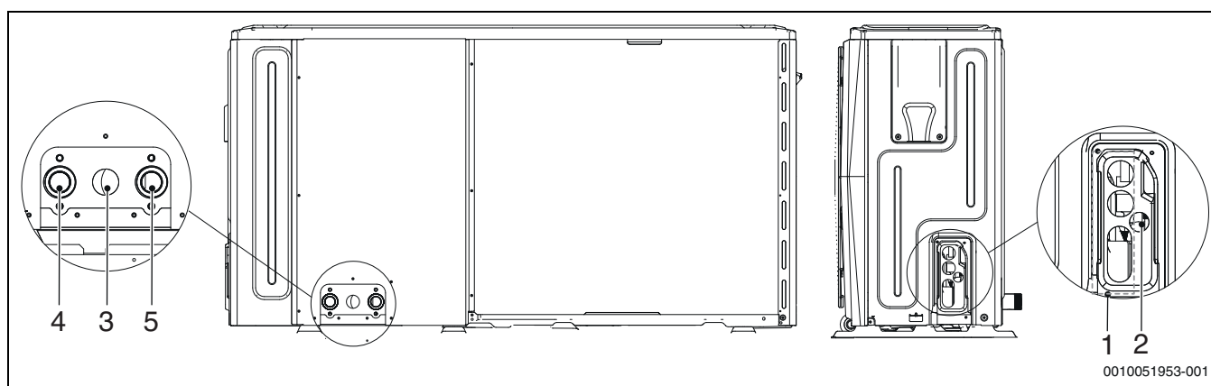
Obr. 64 Velikosti CS2000AWF 4 R-S až CS2000AWF 6 R-S
