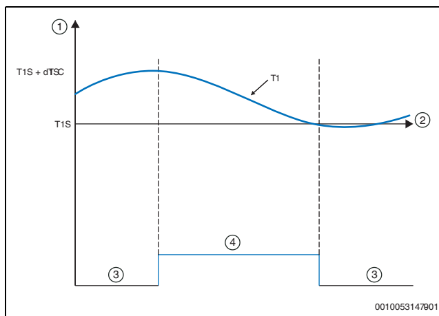
Obr. 122 Režim Chlazení – Teplota přívodu vody ( T_1 )
