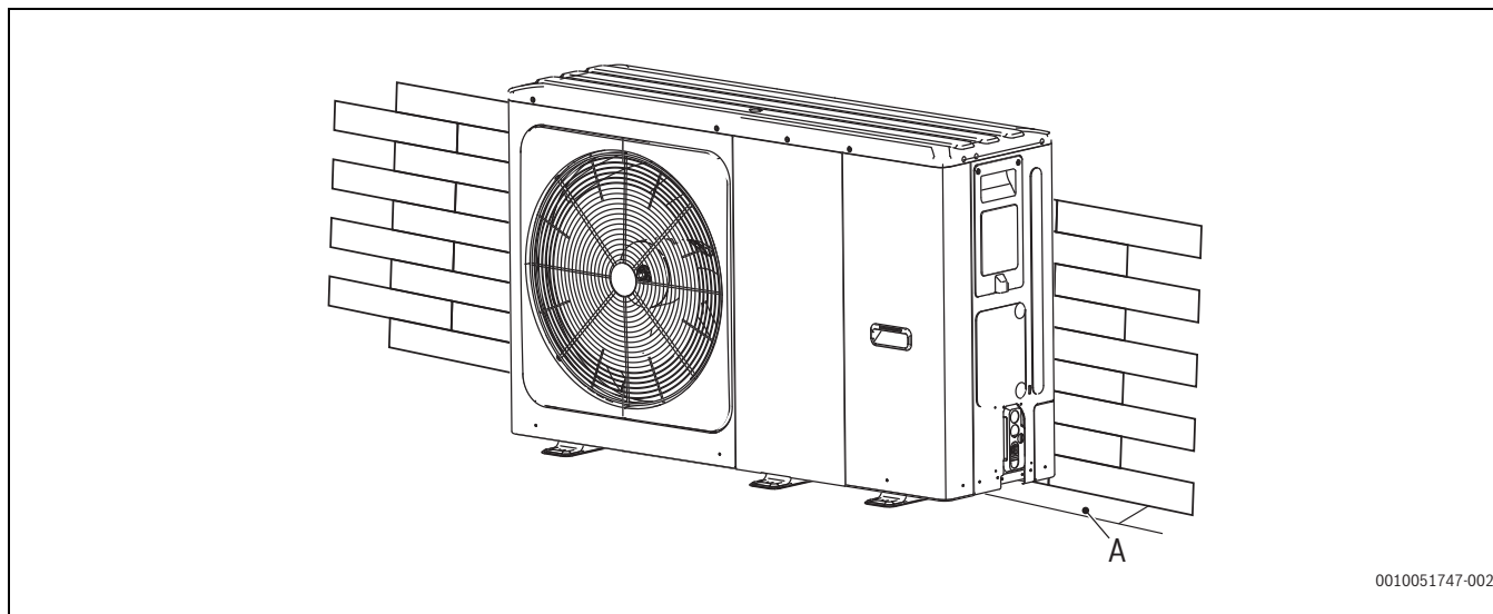
Obr. 35 Standardní instalace modelů CS2000AWF 4 R-S – CS2000AWF 30 R-T
