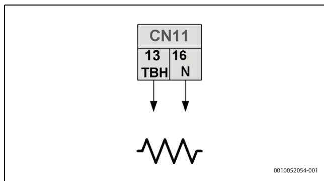
Obr. 79 Konfigurace kabelu přídavného ohřívače na rozhraní HMI, ovládací signál typ 2
