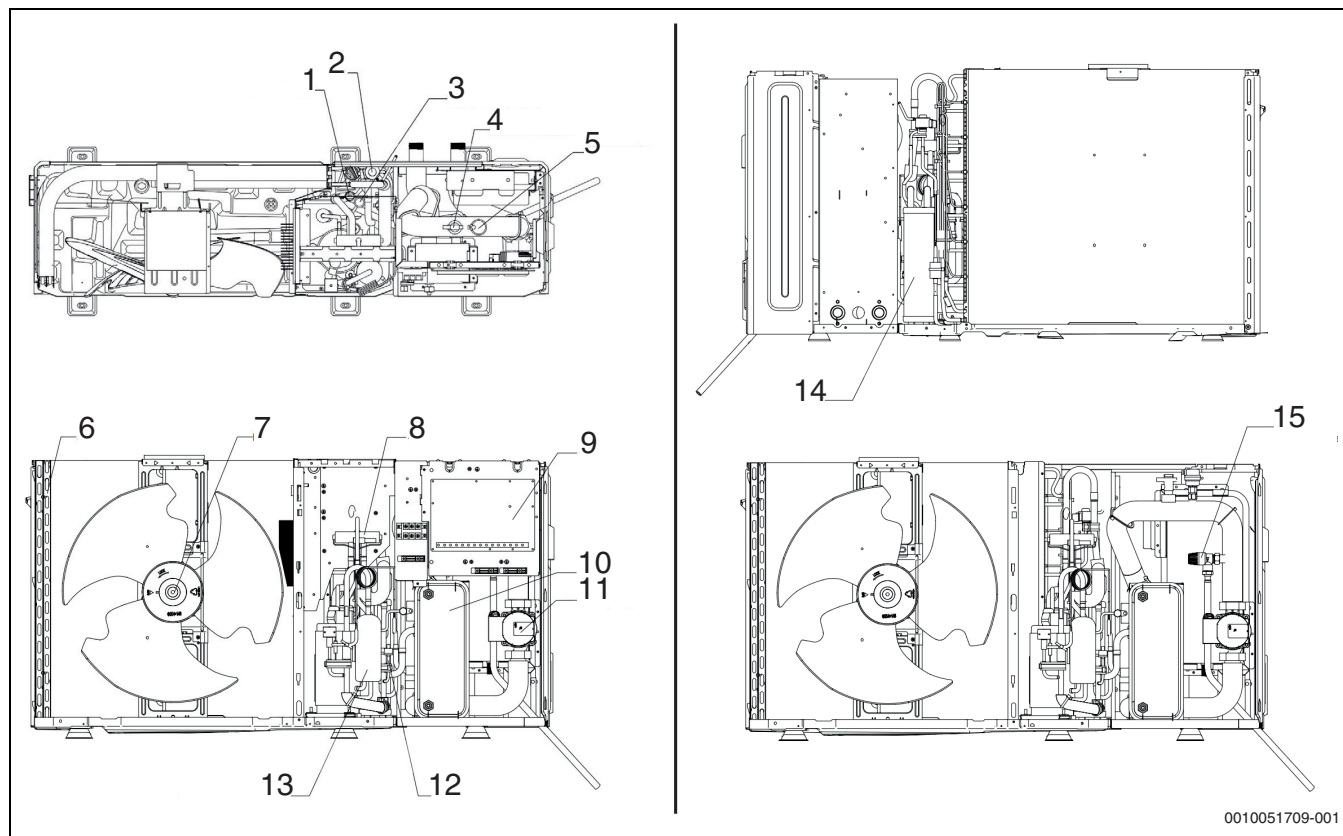
Obr. 2 Velikosti CS2000AWF 4 R-S až CS2000AWF 6 R-S
