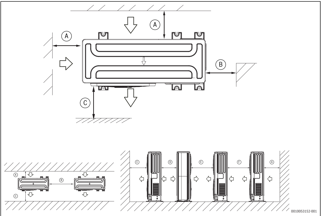
Obr. 36 Minimální vzdálenosti
