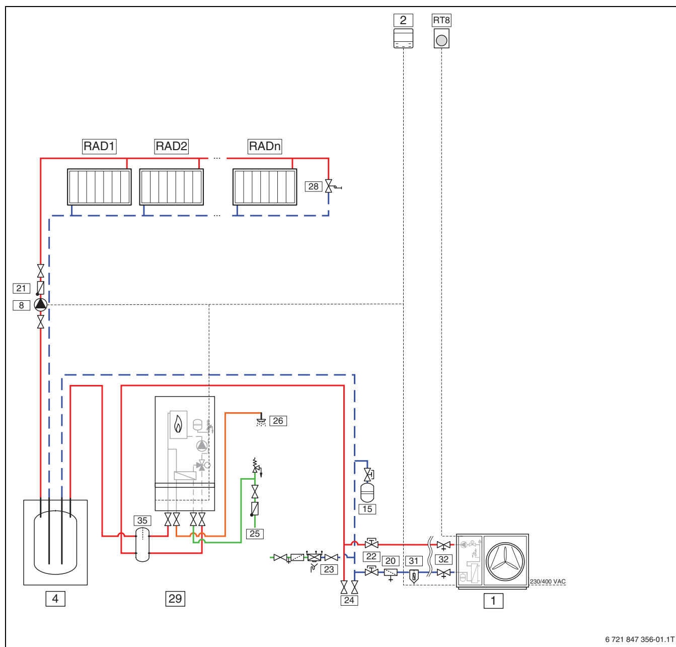
Obr. 26 Venkovní jednotka s nejméně jedním otopným okruhem a externím přídavným ohřívačem (CS2000AWF 4-6 R-S, CS2000AWF 8-10 R-S, CS2000AWF 12-16 R-S/T)
