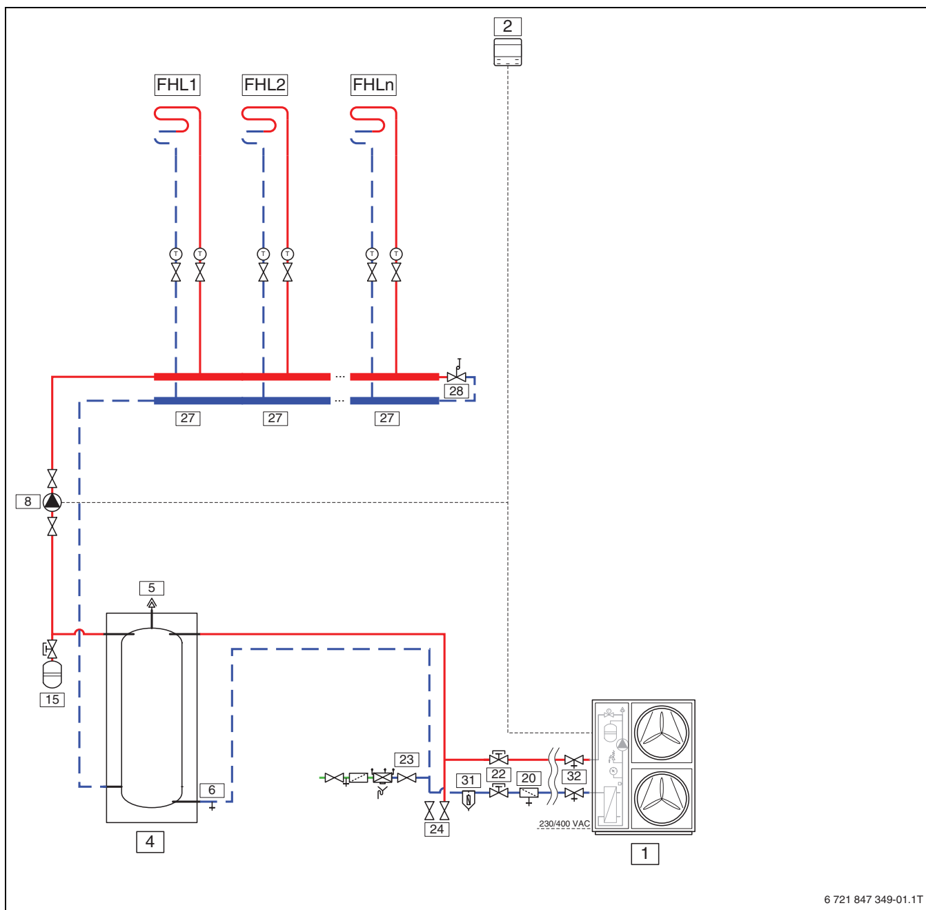
Obr. 19 Venkovní jednotka s nejméně jedním otopným okruhem (CS2000AWF 18-30 R-T)
