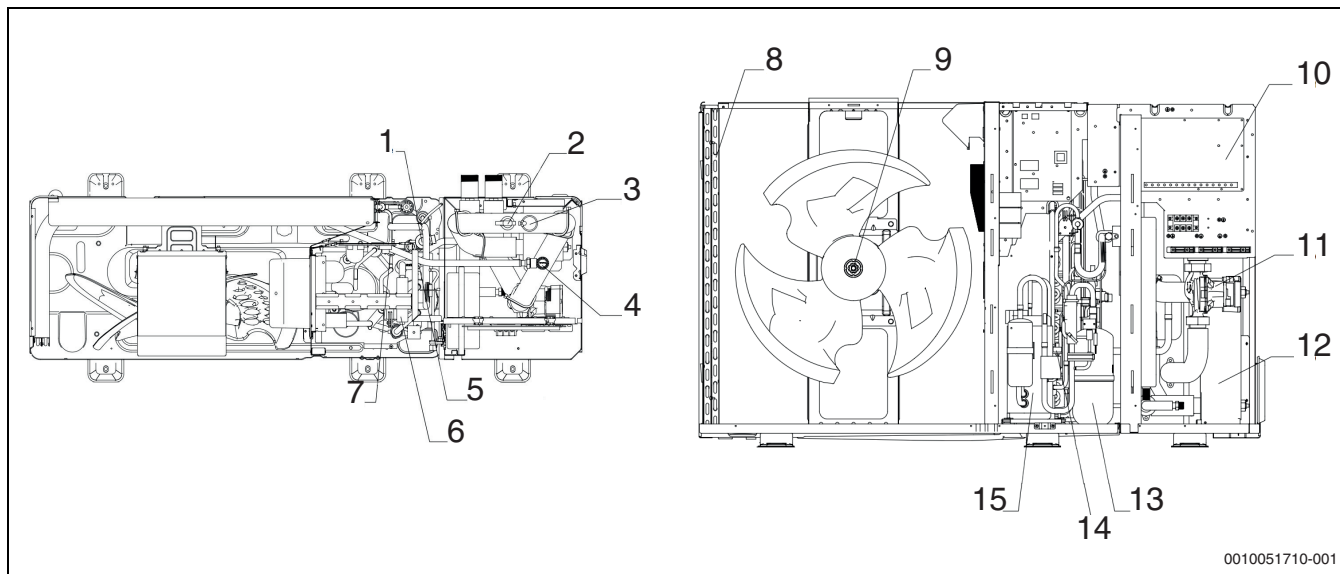
Obr. 3 Velikosti CS2000AWF 8 R-S až CS2000AWF 10 R-S
