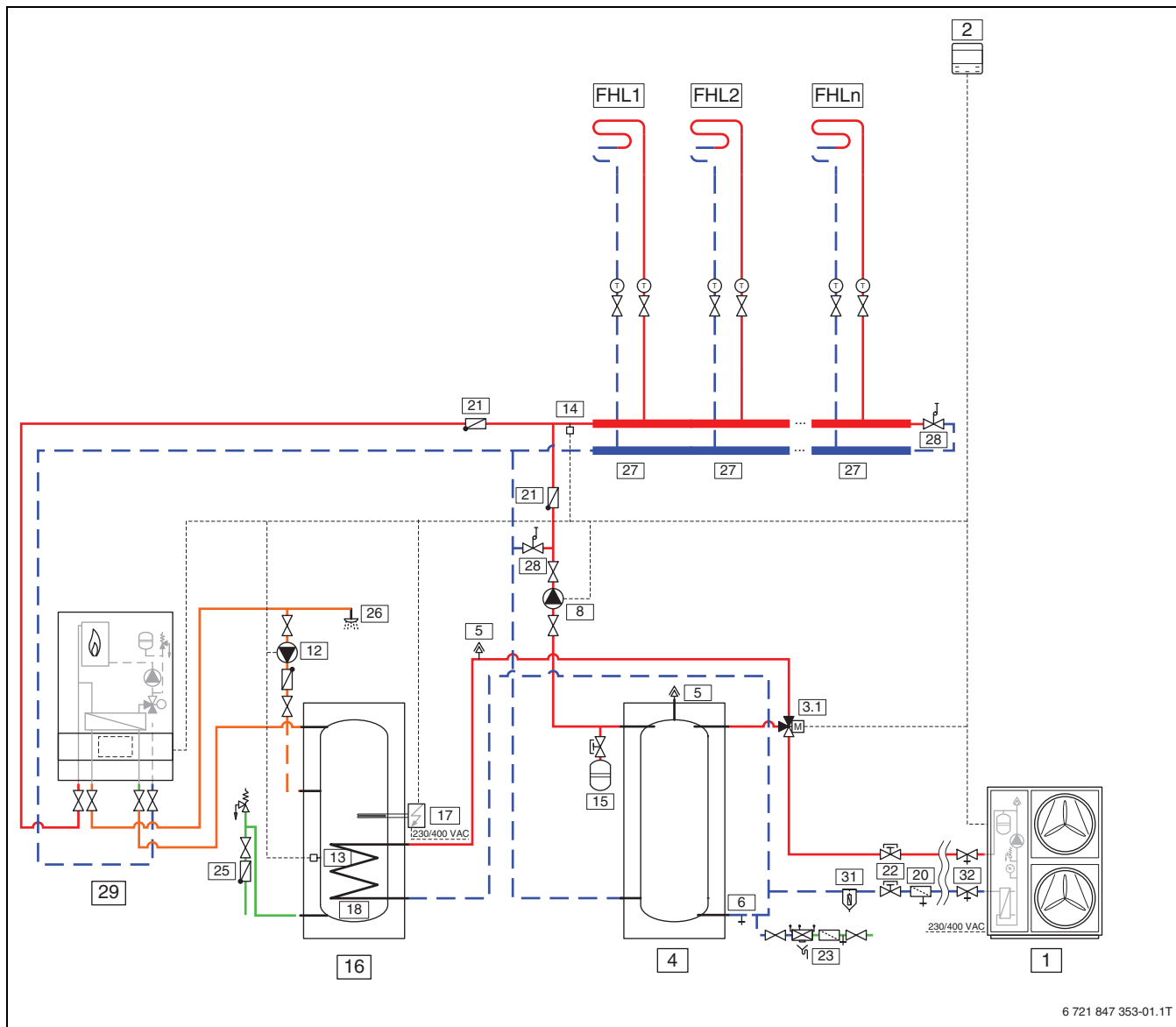
Obr. 23 Venkovní jednotka s nejméně jedním topným okruhem, externím přídavným ohřívačem a zásobníkem TV (CS2000AWF 18-30 R-T)
