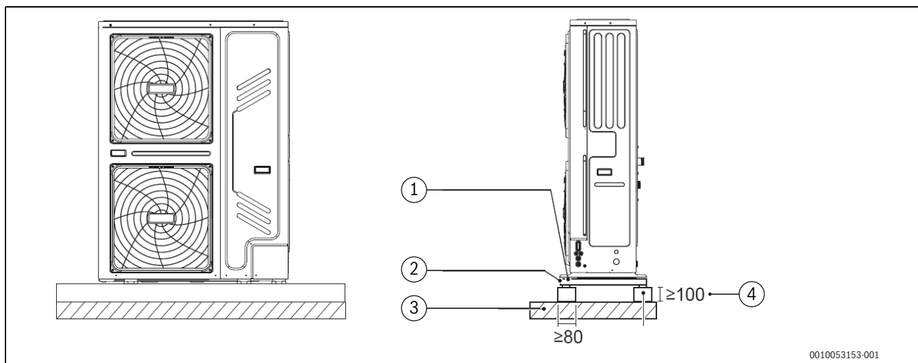
Obr. 43 Zajištění jednotky kotevními šrouby
