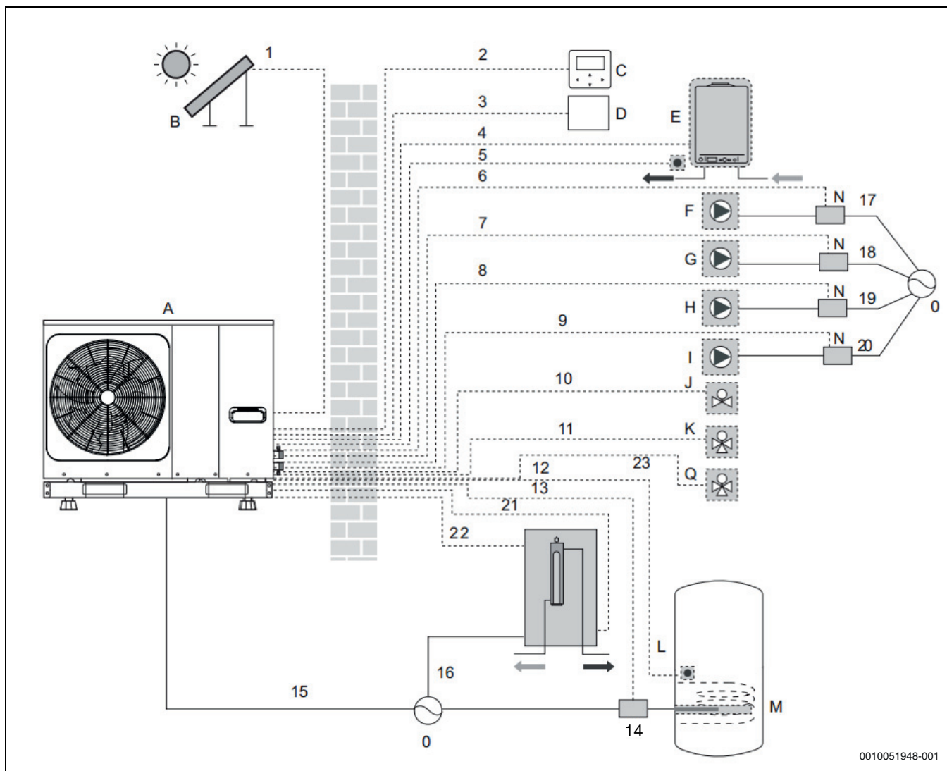
Obr. 61 Obecný diagram
