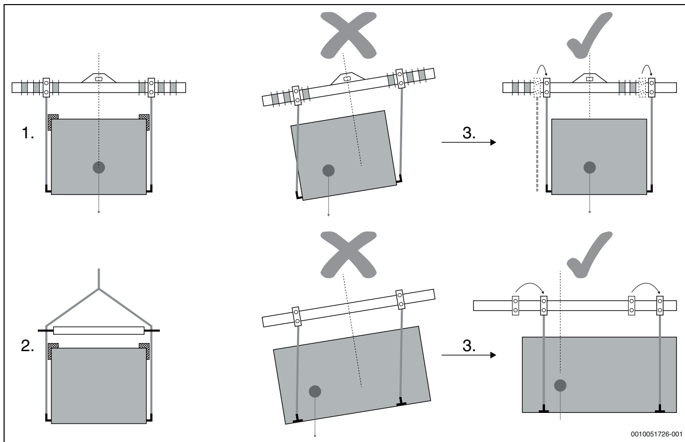
Obr. 29 Zvedání
