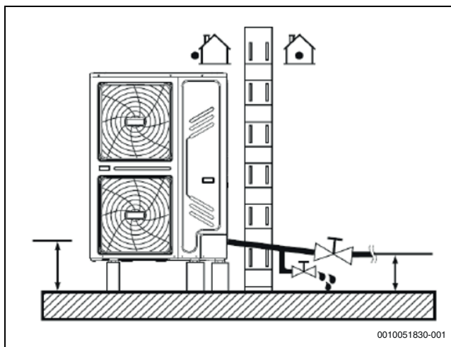
Obr. 54 Ochrana vodního okruhu před zamrzáním
