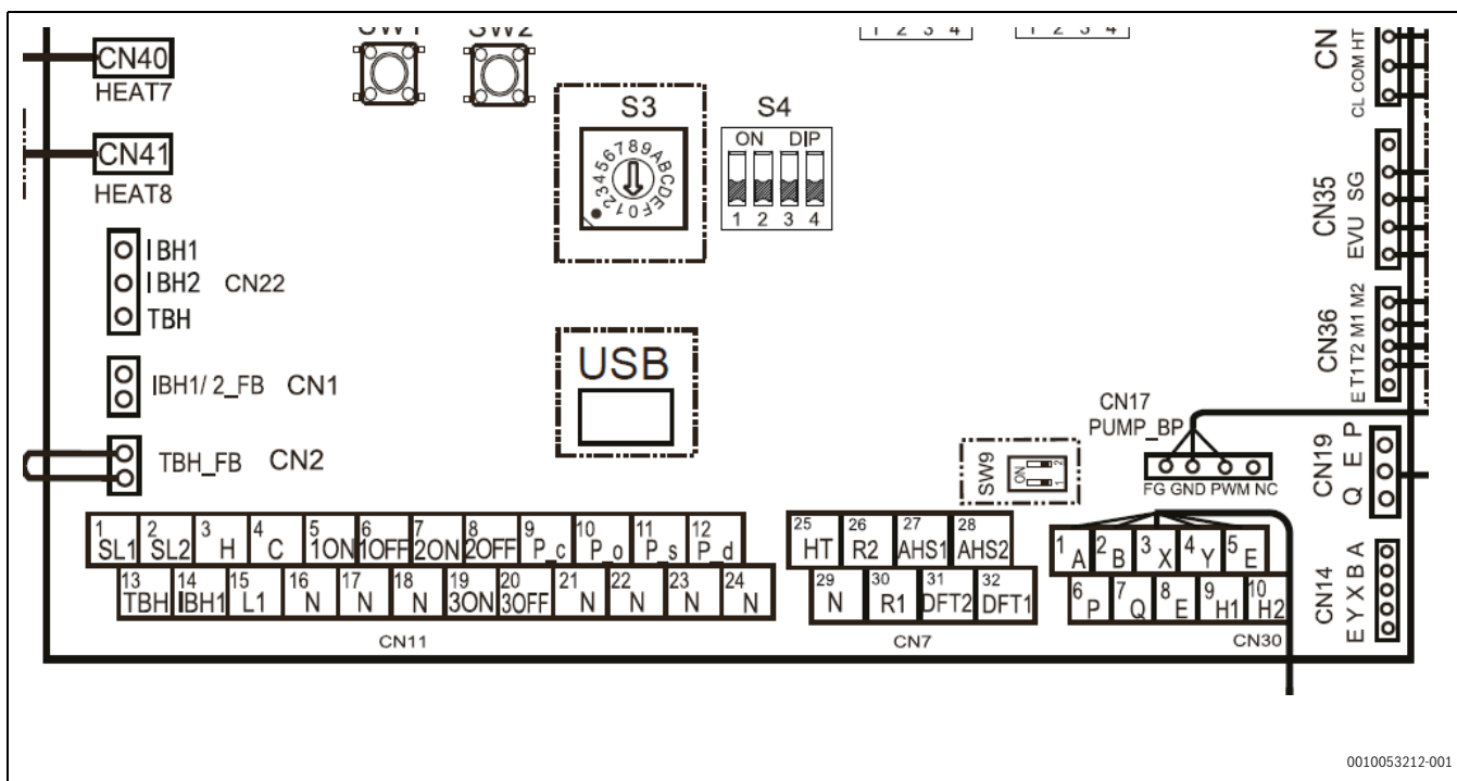
Obr. 73 Připojení svorkovnice
