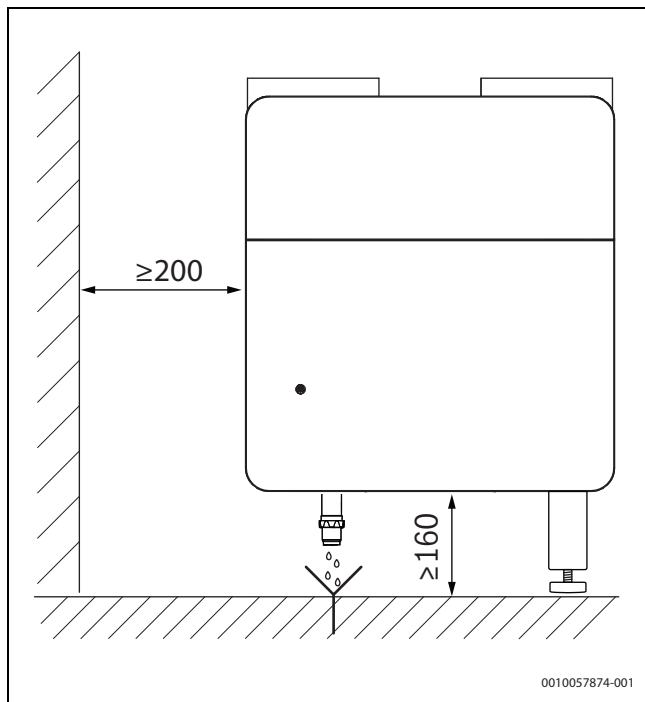
Obr. 44 Minimální vzdálenosti V5001C... se sifonem HRV-MS při montáži na podlahu
