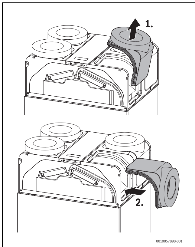
Obr. 20 Vytažení a opětovné nasazení hrdla
