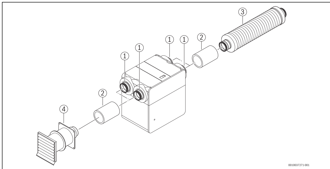
Obr. 54 Připojení systému vzduchových kanálů – varianta 2
