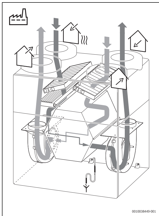
Obr. 28 Varianta B (stav při expedici)
