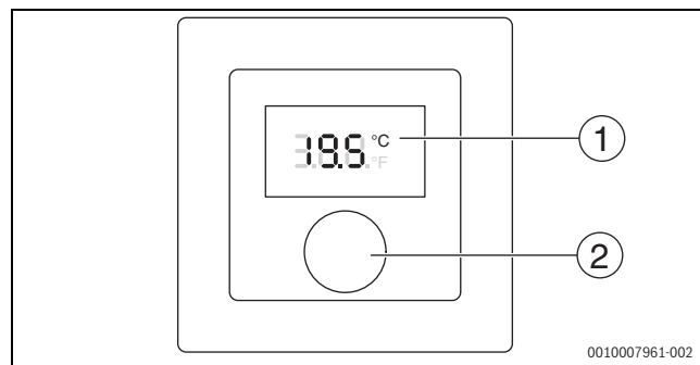
Obr. 56 Ovládací prvky CR 10 H
