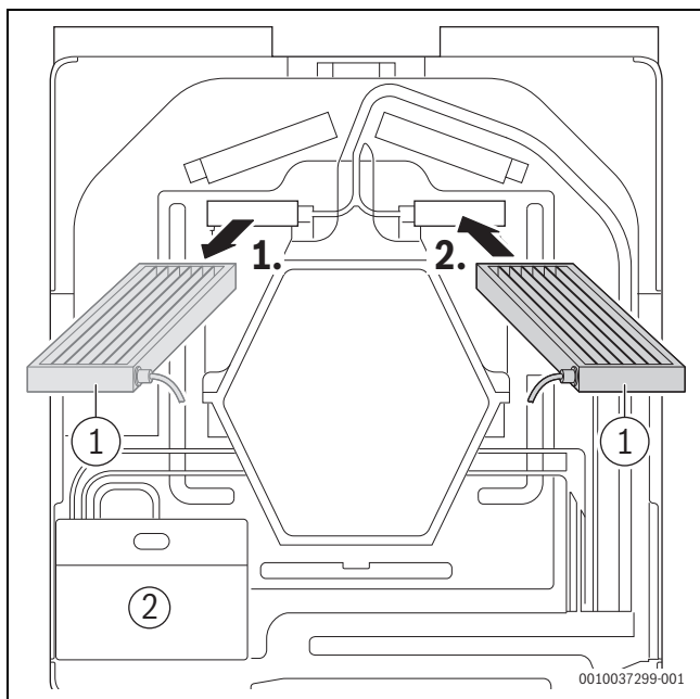
Obr. 30 Přemístění elektrického předehřívacího topného tělesa zleva doprava
