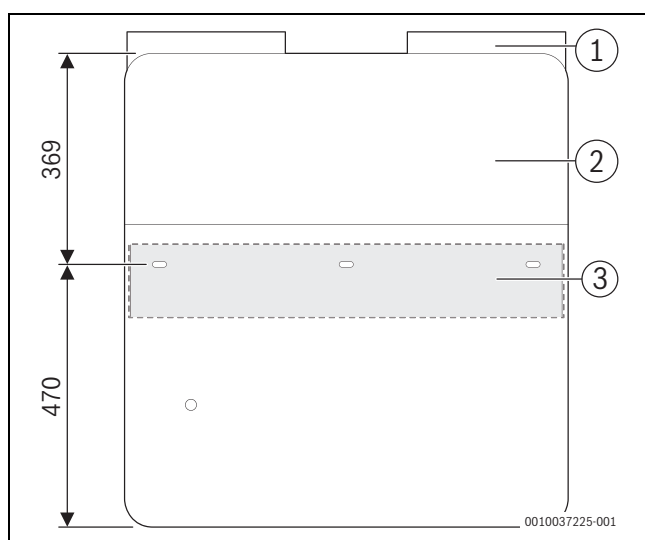
Obr. 34 Montážní rozměry při samostatné instalaci ventilační jednotky
