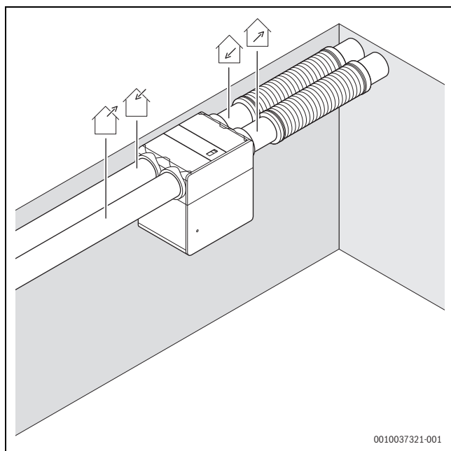
Obr. 51 Varianta 2: Připojky přístroje vodorovně – vedení vzduchu ve variantě B
