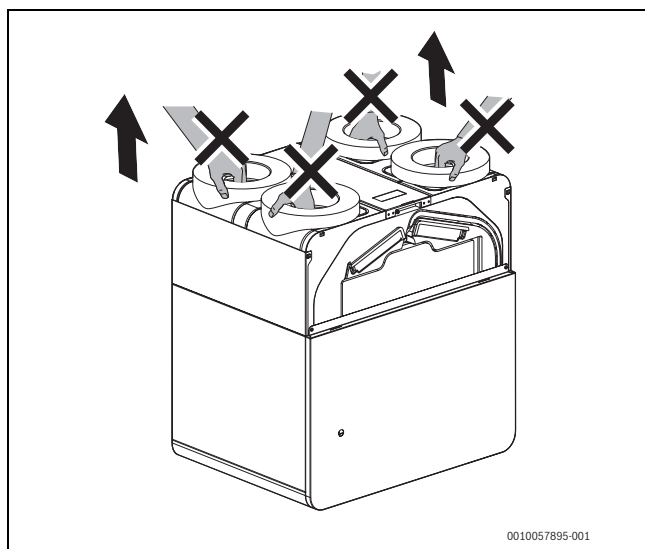
Obr. 16 Nezvedat za přípojovací hrdla
