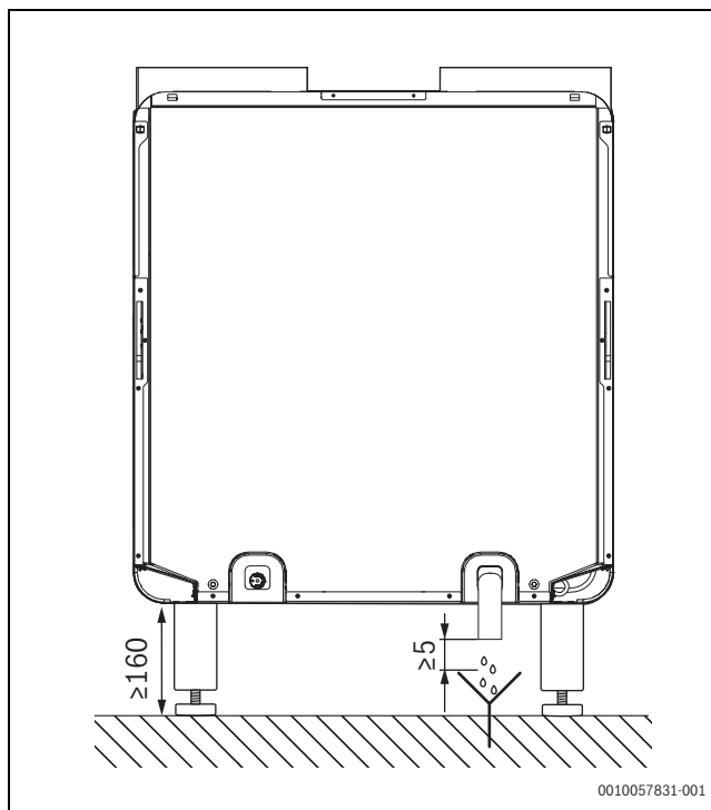
Obr. 38 Minimální vzdálenosti V5001C... s podlahovou konzolou HRV-FMS a připojeným kulovým sifonem HRV-BS nebo membránovým sifonem HRV-MS
