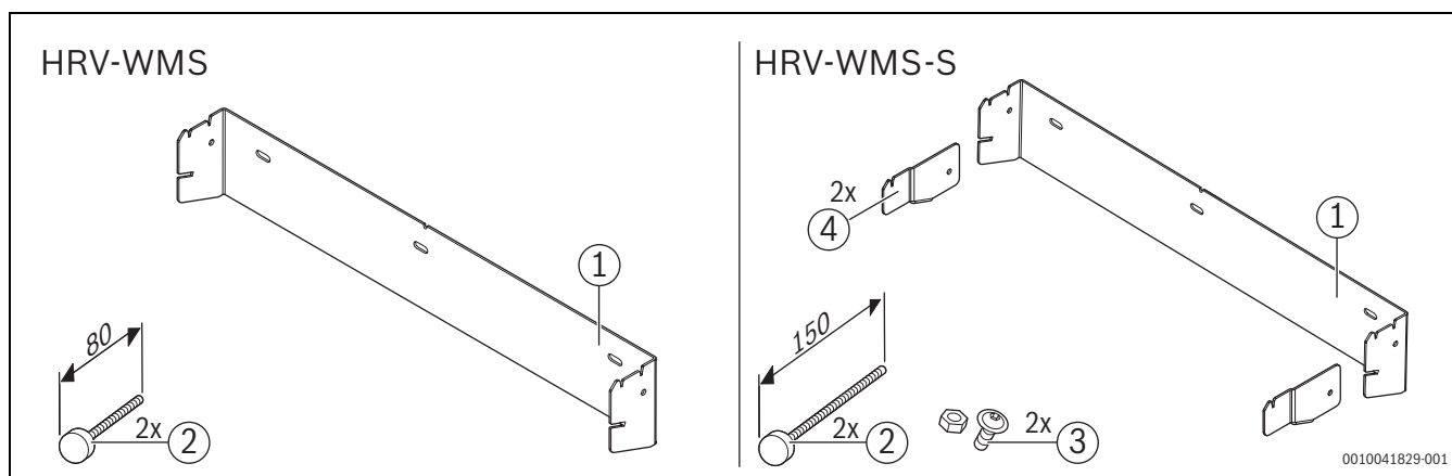
Obr. 33 Rozsah dodávky HRV-WMS/HRV-WMS-S
