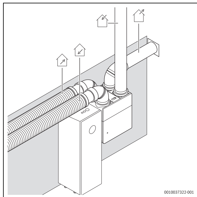
Obr. 52 Varianta 3: Připojky přístroje svisle – vedení vzduchu ve variantě A
