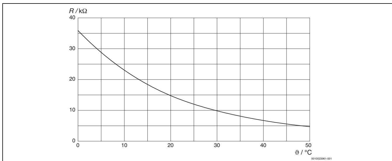
Obr. 74 Charakteristika TV1 (12 K)
