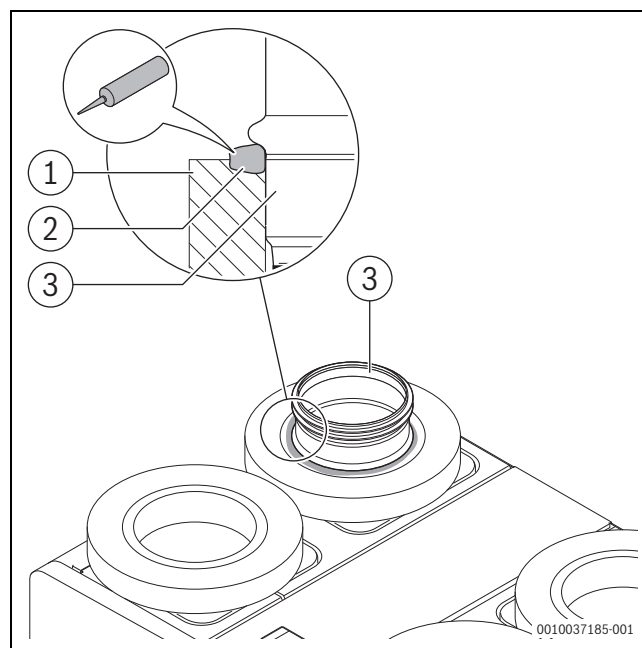
Obr. 48 Utěsnění dvojitého nátrubku FM160
