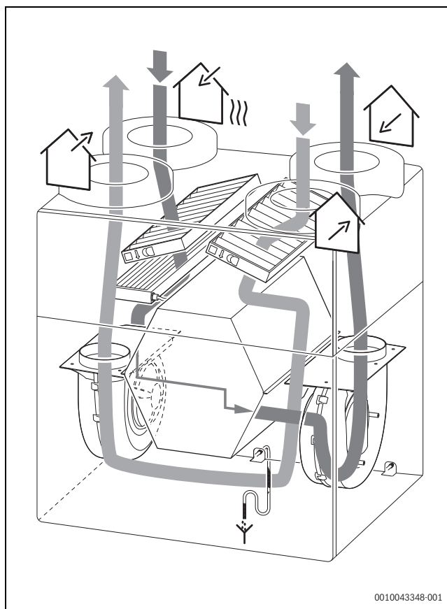
Obr. 12 Příklad vedení vzduchu při provozu obtoku u varianty B
