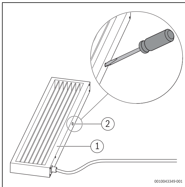
Obr. 69 Reset bezpečnostního omezovače teploty elektrického předehřívacího topného tělesa
