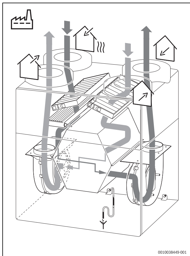
Obr. 10 Stav při expedici: Připojení přístroje na straně vzduchu (varianta B)
