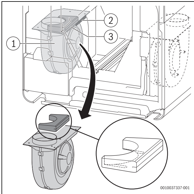
Obr. 67 Vytažení ventilátoru
