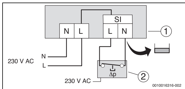
Obr. 61 Připojení hlídače diferenčního tlaku s elektronikou
