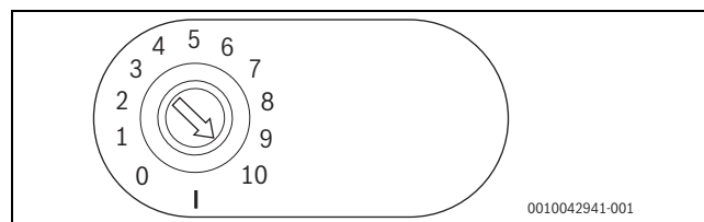
Obr. 72 Kódovací spínač v pozici 10 = autarkní provoz
