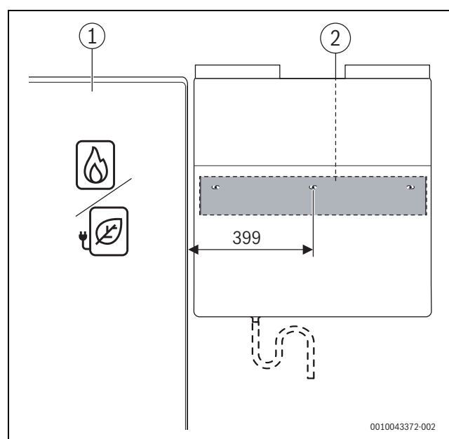
Obr. 36 Vzdálenost zdroje tepla Bosch od V5001C...
