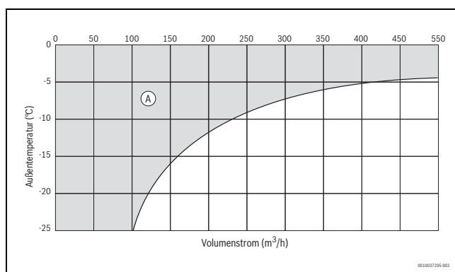
Obr. 13 Maximálně dosažitelný objemový proud
