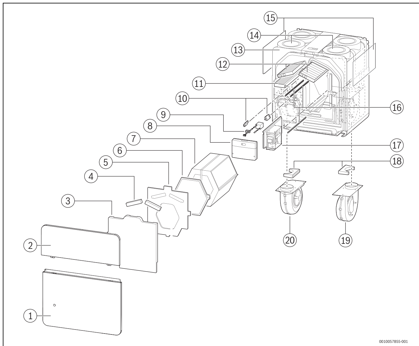
Obr. 8 Přehled výrobku V5001C...
