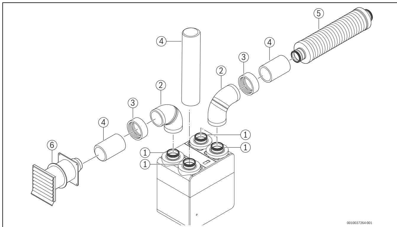
Obr. 53 Připojení systému vzduchových kanálů – varianta 1
