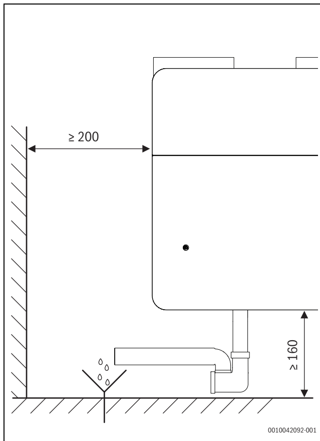
Obr. 42 Minimální vzdálenosti V5001C... se sifonem HRV-BS
