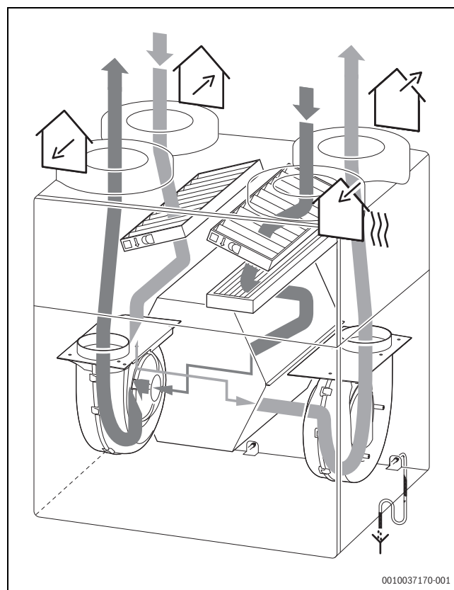
Obr. 11 Připojení přístroje na straně vzduchu (varianta A)
