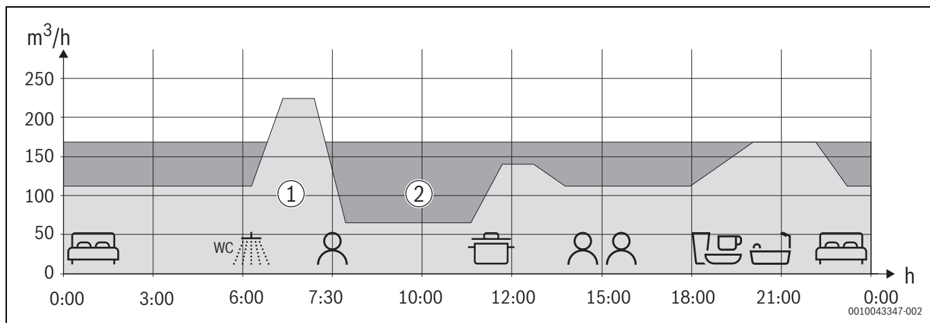
Obr. 14 Příklad porovnání větrání podle potřeby / ručního větrání
