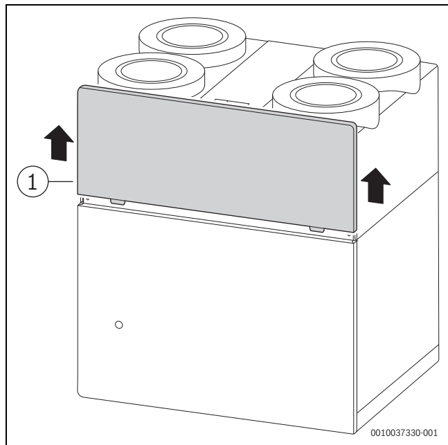
Obr. 24 Sejmутí krycí desky filtru (kov)
