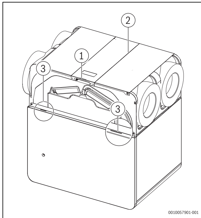
Obr. 23 Otvory pro spony krycí desky filtru
