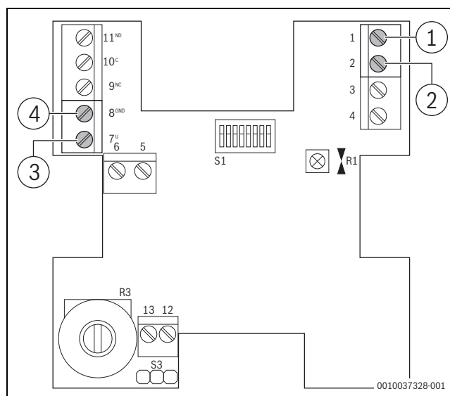
Obr. 59 Interní elektrické připojky CS/VS-R
