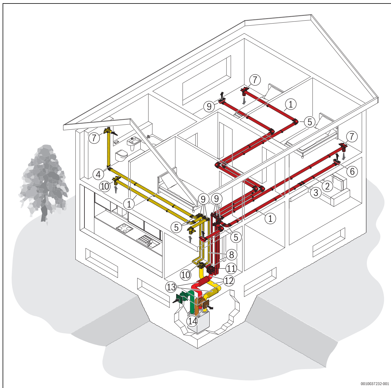
Obr. 15 Příklad systému s příslušenstvím
