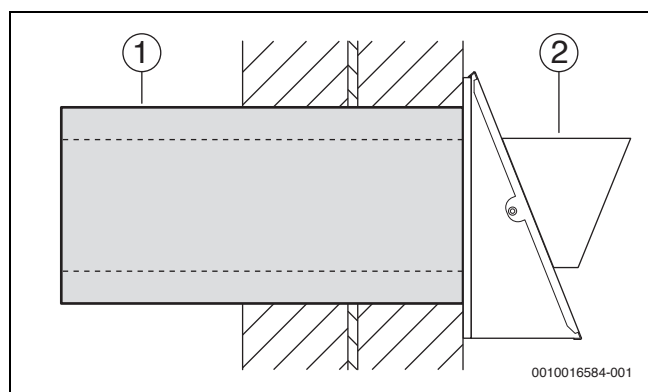
Obr. 46 Izolace trubek
