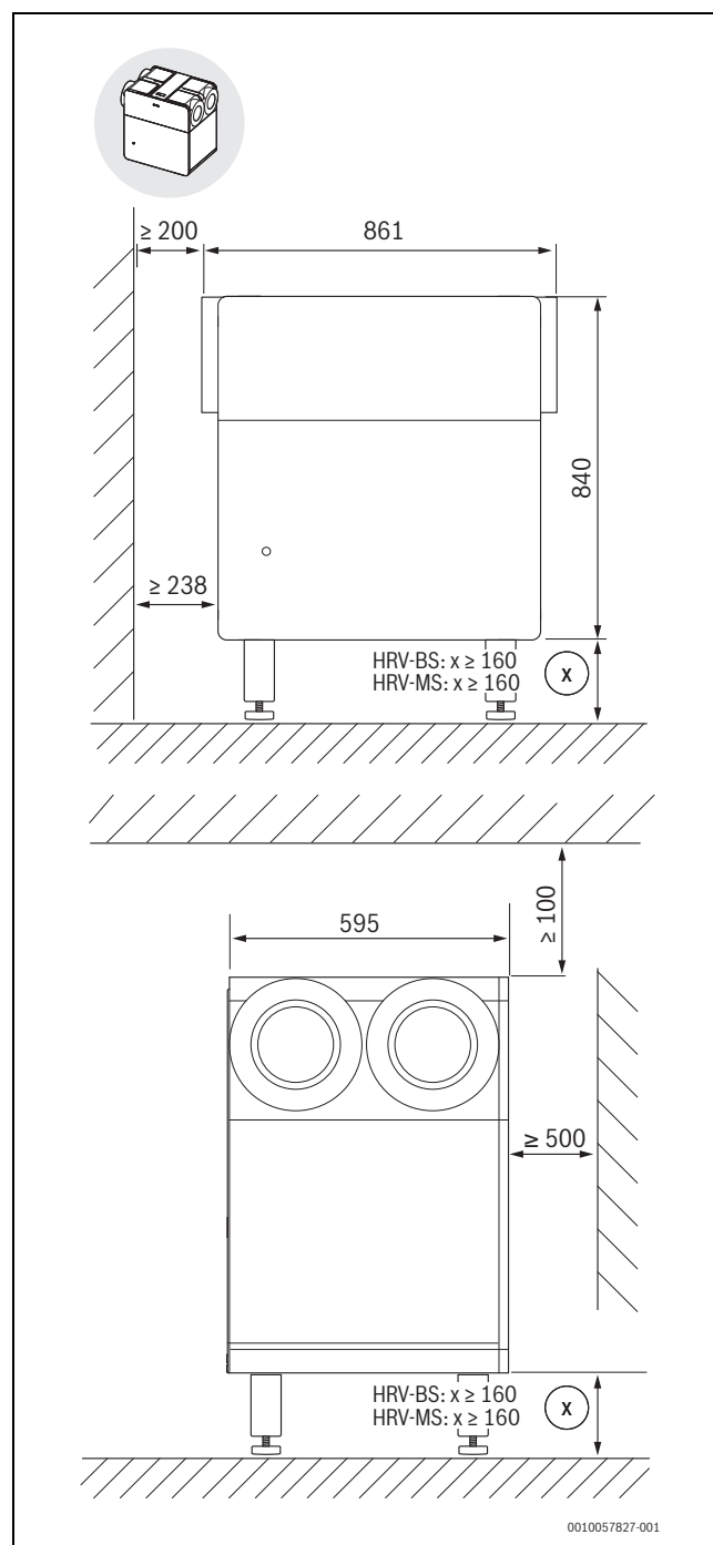
Obr. 6 Rozměry a minimální vzdálenosti při instalaci na podlahu V5001C... – minimální vzdálenosti, pokud je připojovací hrdlo nainstalováno vodorovně
