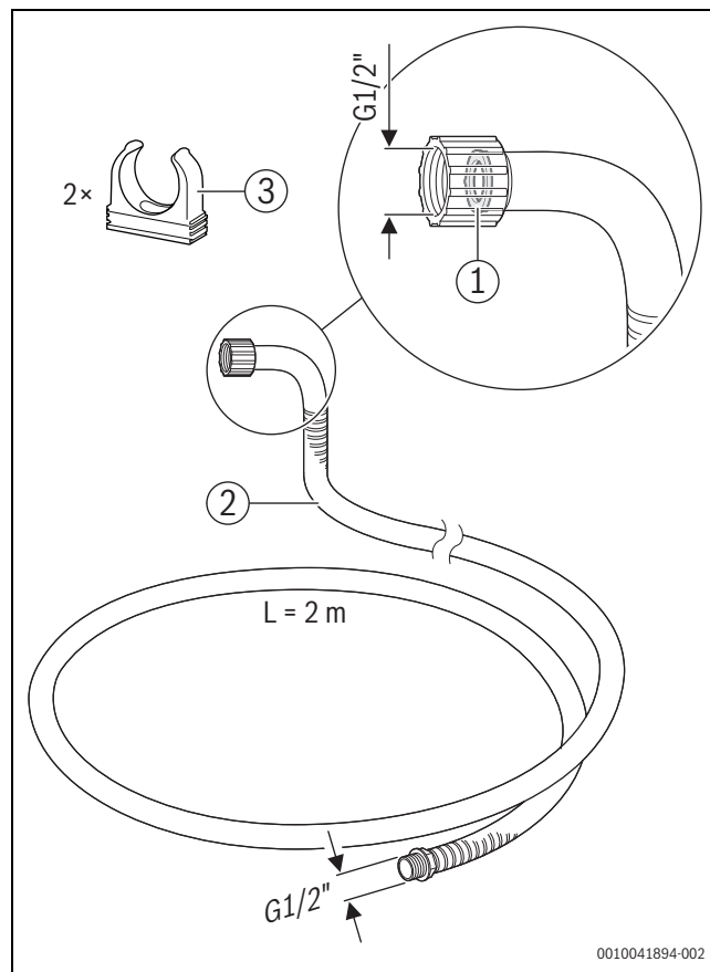
Obr. 39 Sada pro připojení flexibilního sifonu
