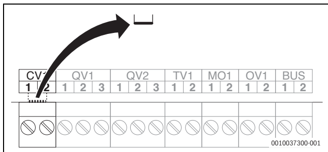
Obr. 31 Odstranění můstku
