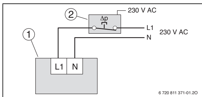
Obr. 62 Připojení hlídače diferenčního tlaku v elektrickém vedení
