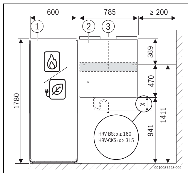
Obr. 35 Montážní rozměry v systému se zdrojem tepla Bosch
