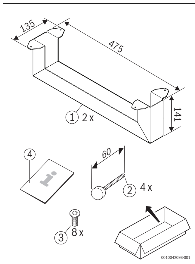
Obr. 37 Rozsah dodávky HRV-FMS
