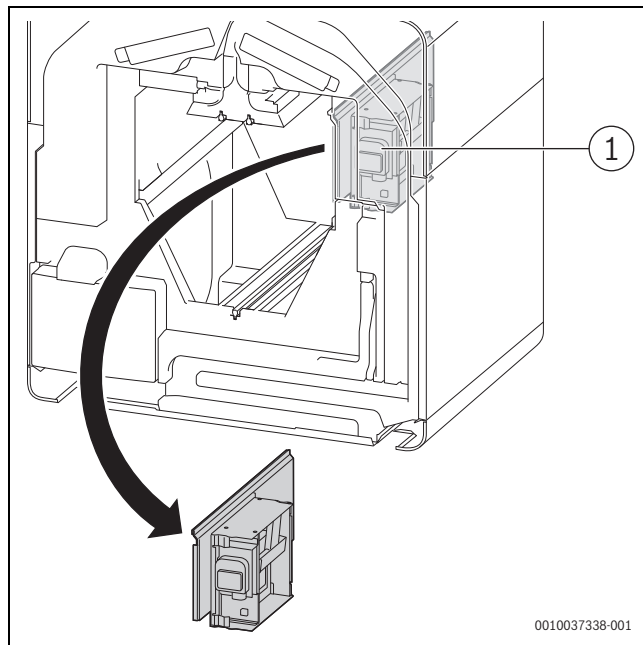
Obr. 68 Vyjmutí obtoku
