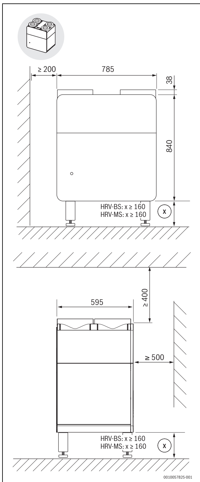
Obr. 5 Rozměry a minimální vzdálenosti při instalaci na podlahu V5001C... – minimální vzdálenosti, pokud je připojovací hrdlo nainstalováno svisle
