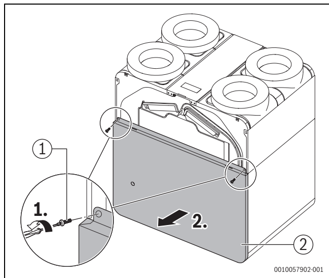
Obr. 25 Povolení šroubů a sejmутí krycí desky základního tělesa z EPP (kov)
