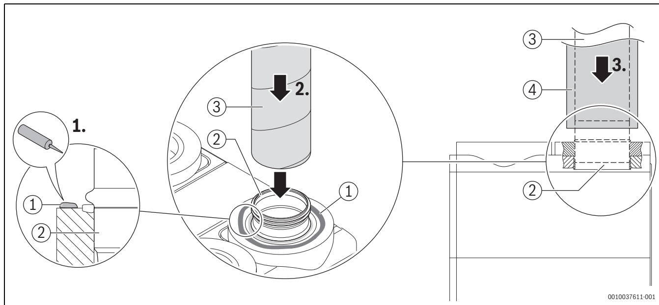
Obr. 49 Konstrukční uspořádání přípojky vzduchové trubky
