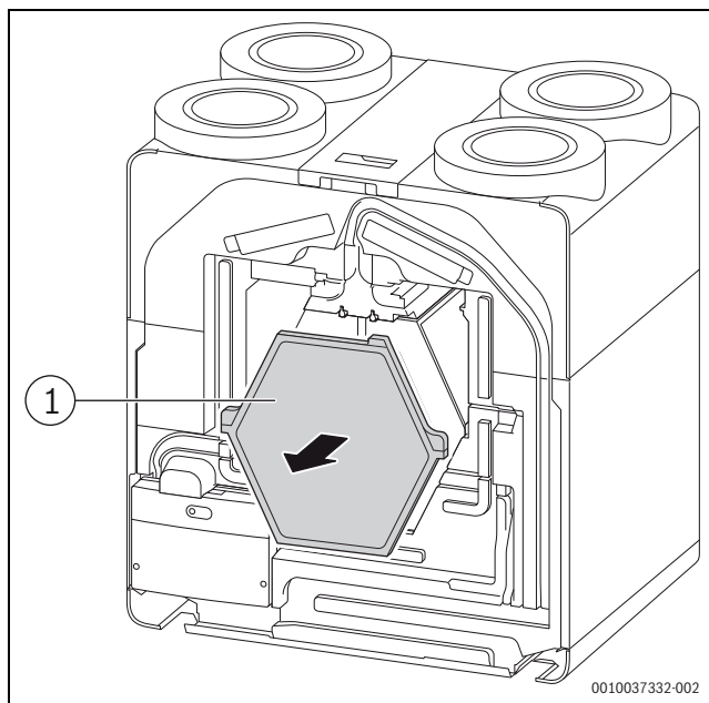
Obr. 27 Sejmутí distanční vložky z EPP
