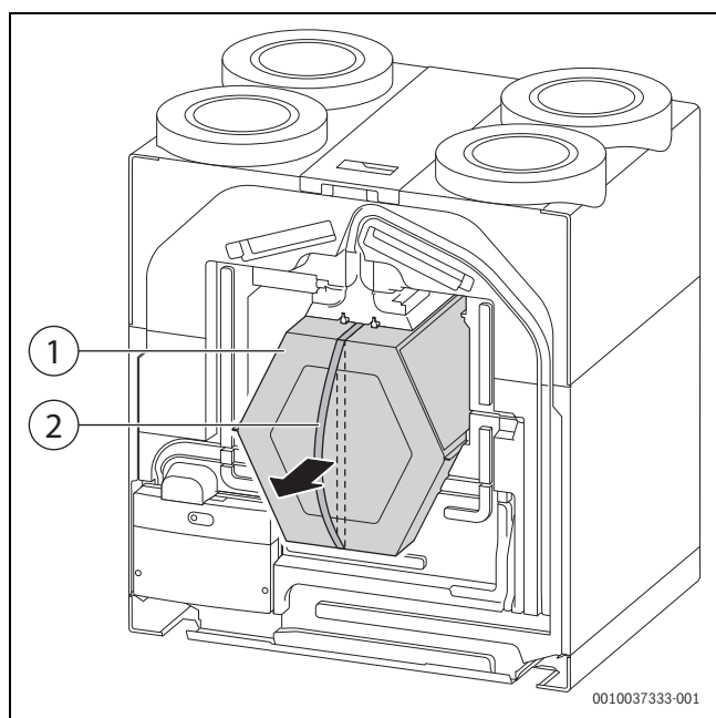
Obr. 66 Vytažení výměníku tepla
