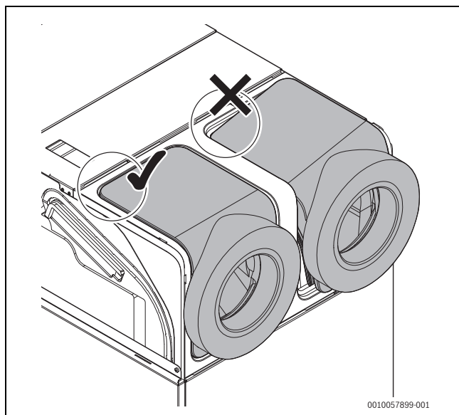
Obr. 21 Správné usazení připojovacích hrdel
