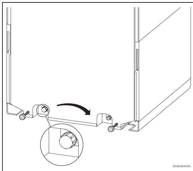
Obr. 32 Přestavba odvodu kondenzátu (pohled zezadu na přístroj)
