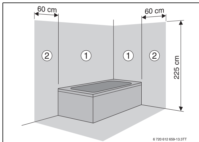
Obr. 29 Ochranné úseky
