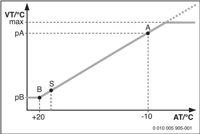
Obr. 36 Ekvitermní křivka
