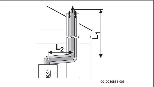
Obr. 8 Koncentrický systém odvodu spalin podle C 33x v šachtě
