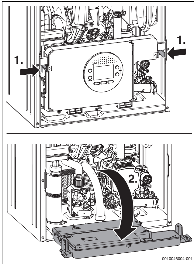
Obr. 32 Sklopení elektroniky směrem dolů
