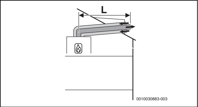
Obr. 7 Horizontální koaxiální systém odvodu spalin podle C 13x přes střechnu
