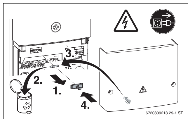
Obr. 44 Výměna pojistky
