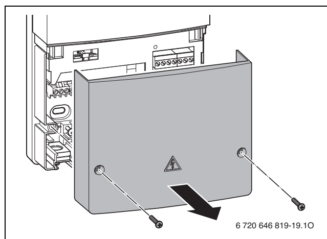
Obr. 31 Otevření modulu
