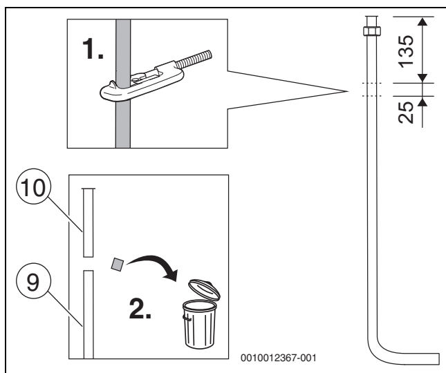
Obr. 20 Příprava dlouhého přípojovacího potrubí
