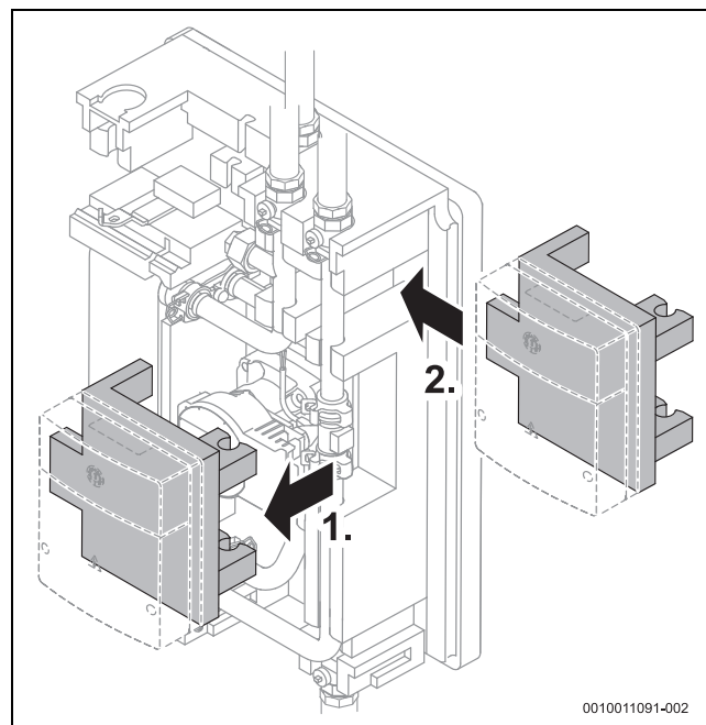
Obr. 40 Změna zapojení modulu pro účely údržby
