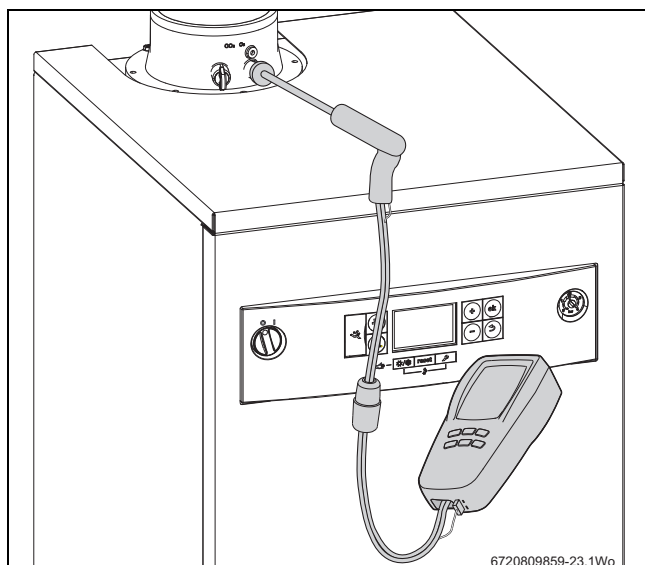
Obr. 47 Test těsnosti odtahu spalín
