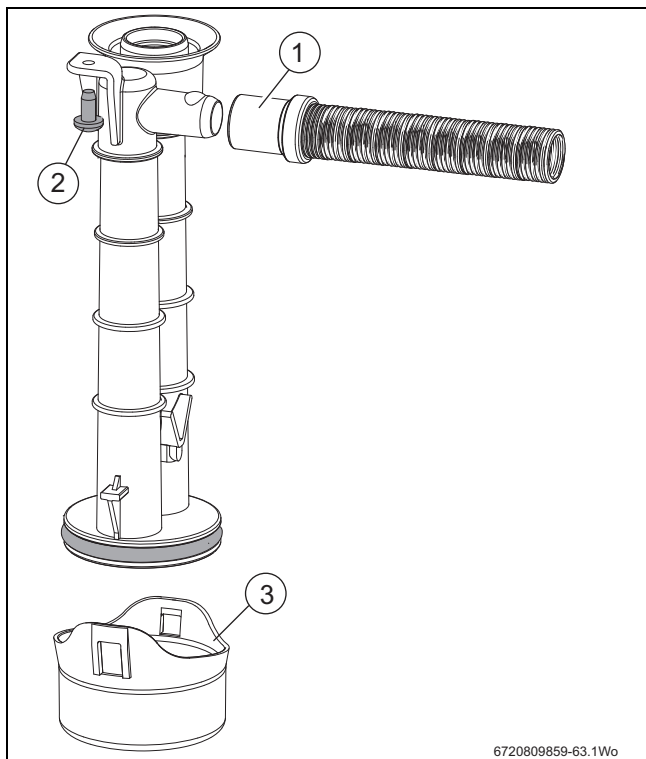
Obr. 66 Sifon kondenzátu
