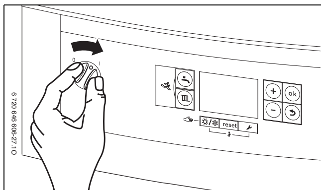
Obr. 33 Hlavní vypínač
