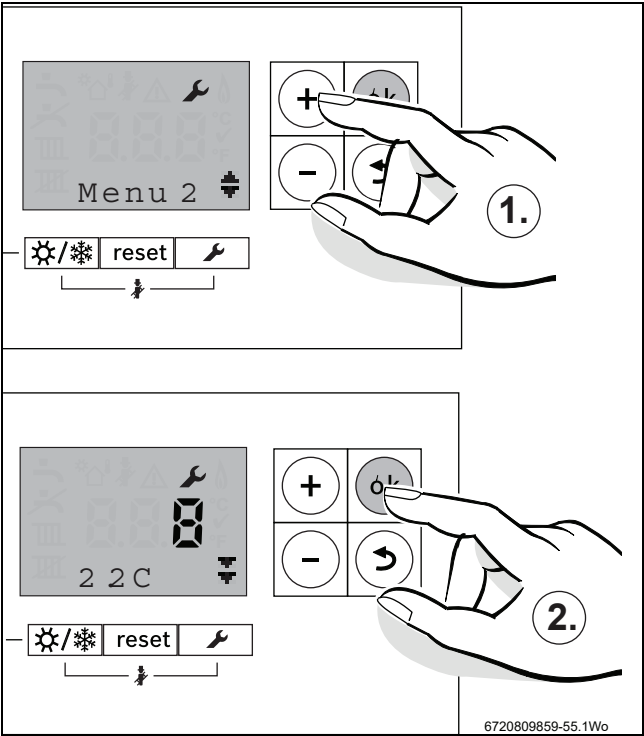
Obr. 73 Výběr Menu 2
