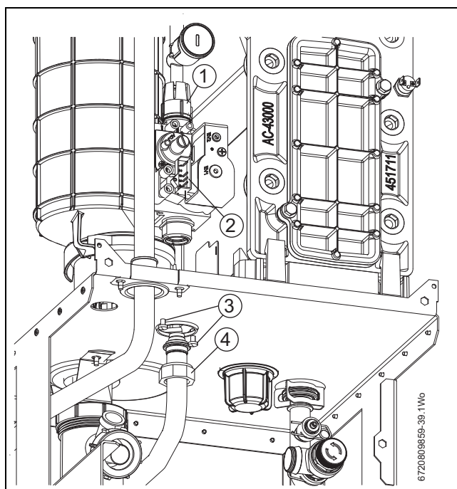
Obr. 67 Plynová armatura
