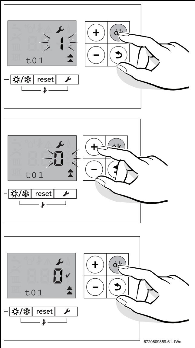
Obr. 79 Test resetování
