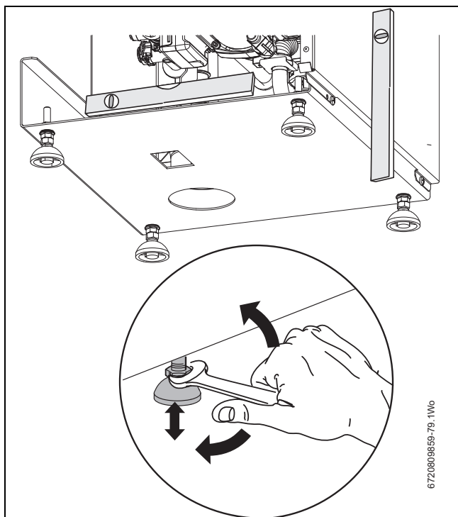
Obr. 16 Vyrovnání kotle
