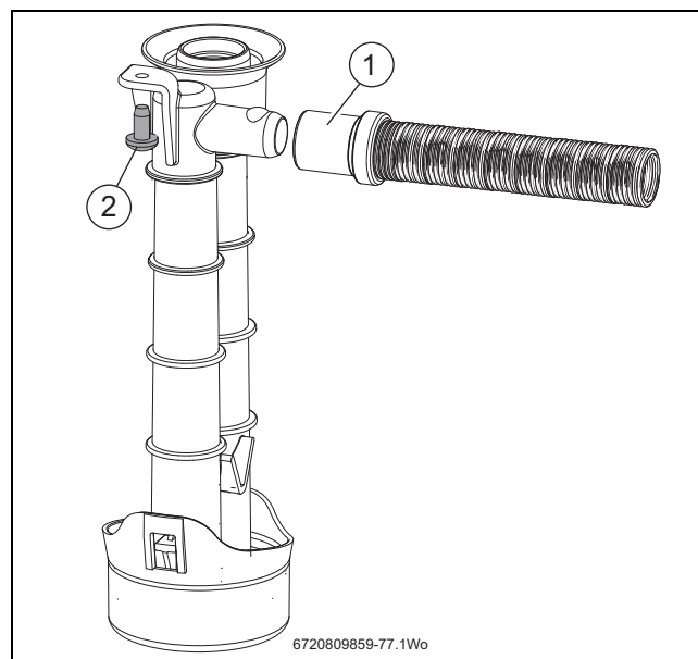
Obr. 12 Sifon kondenzátu
