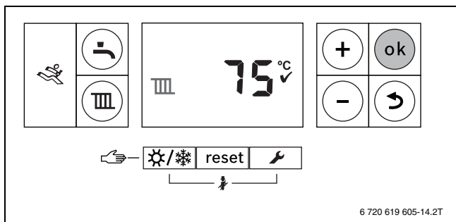
Obr. 5 Displej režimu Vytápění
