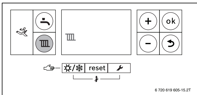
Obr. 4 Displej Vytápění
